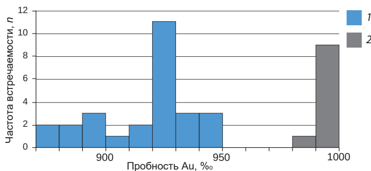
Рис. 11. Пробность золота месторождения Южные Ашалы: типы руд: 1 – золото-сульфидный, 2 – золото-сульфидно-кварцевый; n = 42
