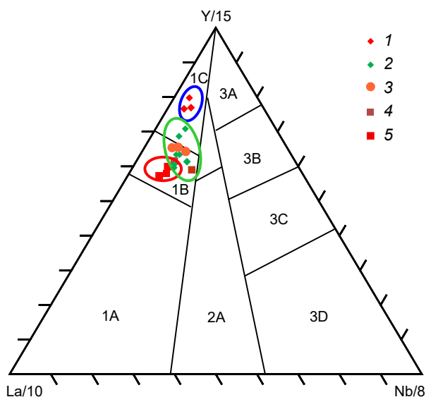
Рис. 2. Дискриминационная диаграмма La-Y-Nb [13] для верхнеюрских–нижнемеловых базальтов Удско-Мургаляского вулканогенного пояса и Охотско-Тайгонской палеоостроводужной системы:
