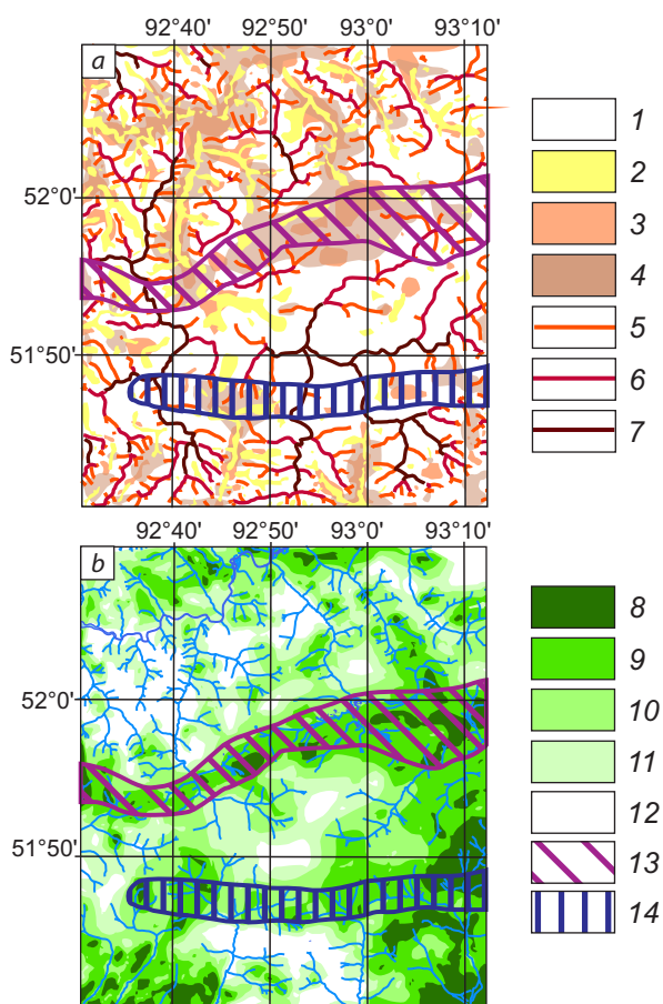
Рис. 4. Карты разностей уровней соседних вершинных поверхностей (а) и вершинных и базисных поверхностей 2-го порядка (b):
