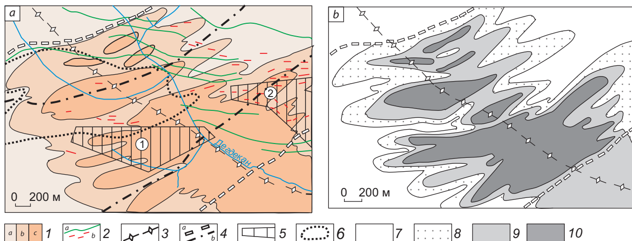
Рис. 4. Литолого-структурная схема участка пересечения Тенькинской антиклинали Дегдеканской зоной складчатых дислокаций (а) и схема распределения C_{org.} в сланцах пионерской свиты (b):
