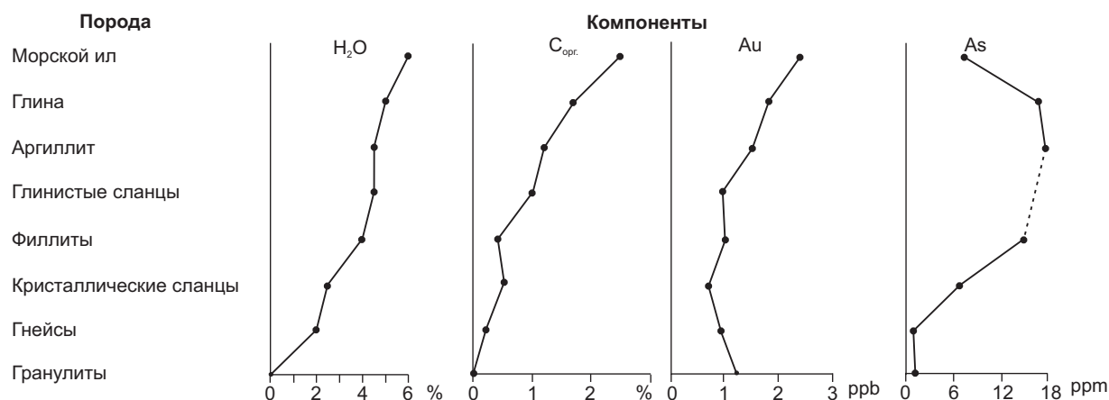
Рис. 1. Поведение C_{\text{орг.}} , Au, H_2O и As в процессе литификации и метаморфизма осадочных пород [24]
