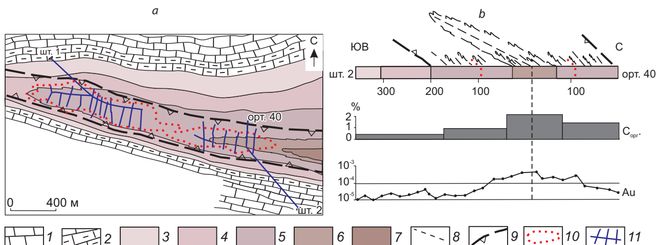
Рис. 9. Геолого-структурный план месторождения Сухой Лог (а), штольневый горизонт, и распределение C_{org} и Au в филлитовидных сланцах сечения шт. 2 – орт. 40 (б) (составлен по материалам (С. Д. Шер и др., 1977)):
