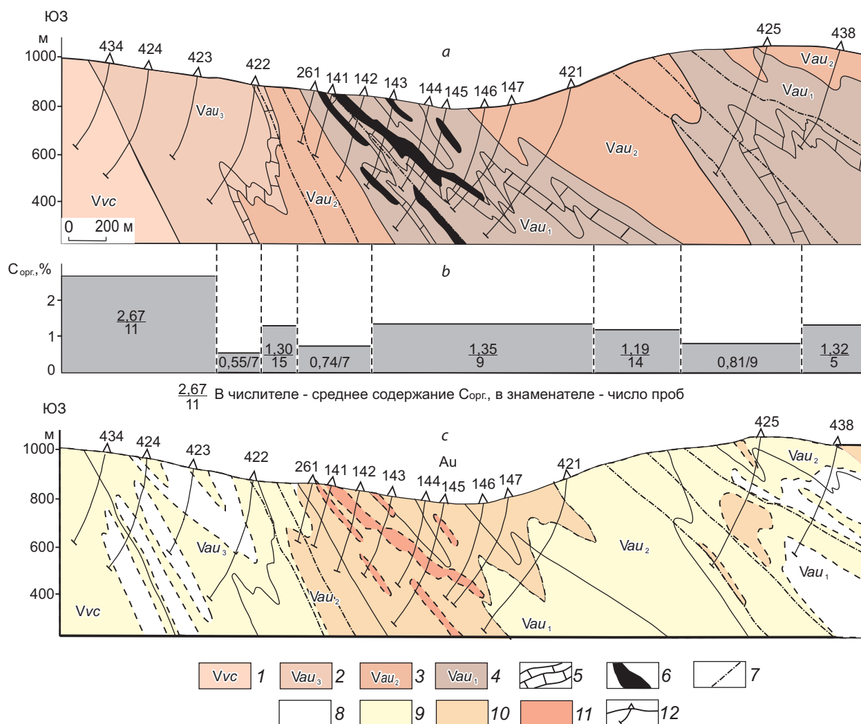
Рис. 8. Геологический разрез по линии БЛ +9 (а), распределение содержаний C_{орг} (b) и золота (с) в сланцах аунакитской свиты:
