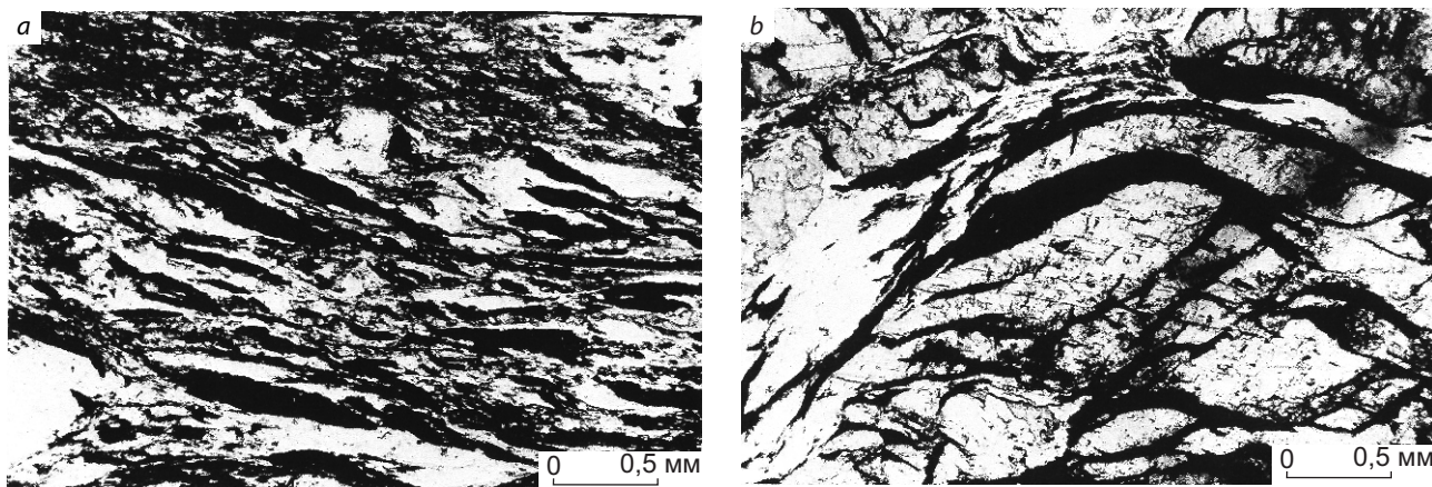
Рис. 10. Линзовидные сегрегации УВ (чёрное) в ассоциации с тонкозернистым кварцем в метаалевролитах (а); чешуйчатые, прожилковидные сегрегации УВ (чёрное), тонкозернистого кварца (белое) в перекристаллизованном карбонате (серое) (b)
