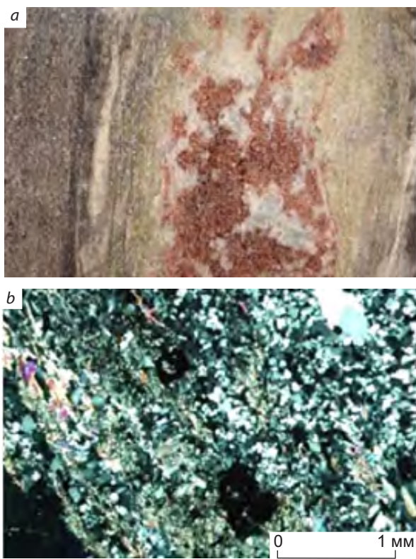
Рис. 15. Кварц-серцит-эпидот-гранатовый скарноид:
