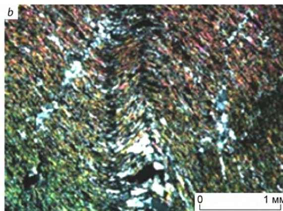
Рис. 7. Углеродсодержащие алевроаргиллиты:
