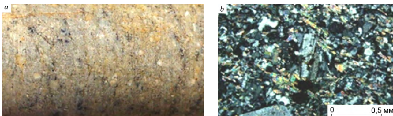
Рис. 11. Риодацит; порфировые выделения плагиоклаза в рассланцованной кварц-полевошпат-мусковитовой основной массе:
