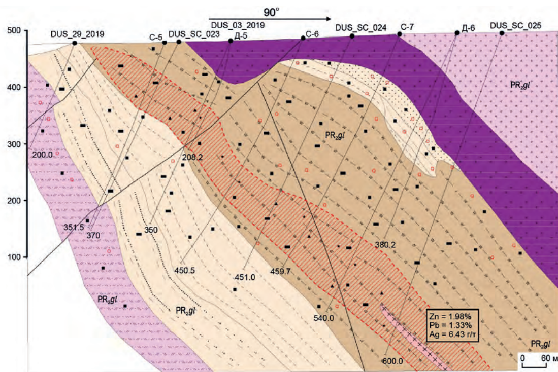
Рис. 4. Схематический литолого-фациальный разрез по профилю 10 (IV):
