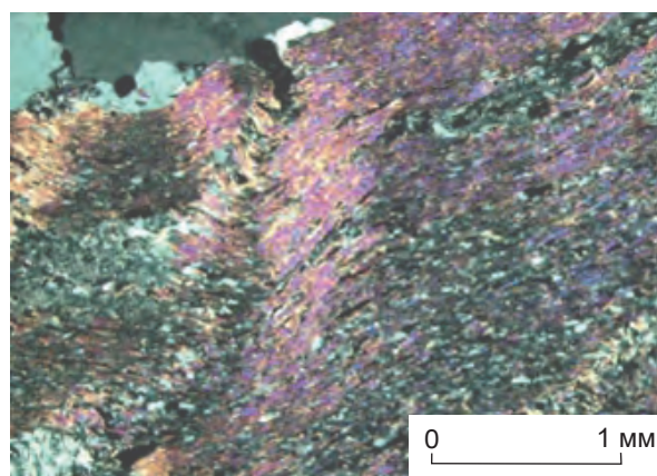
Рис. 13. Алевроаргиллит, превращённый в кварц-мусковитовый сланец с пloyчатой микротекстурой; николи скрещены
