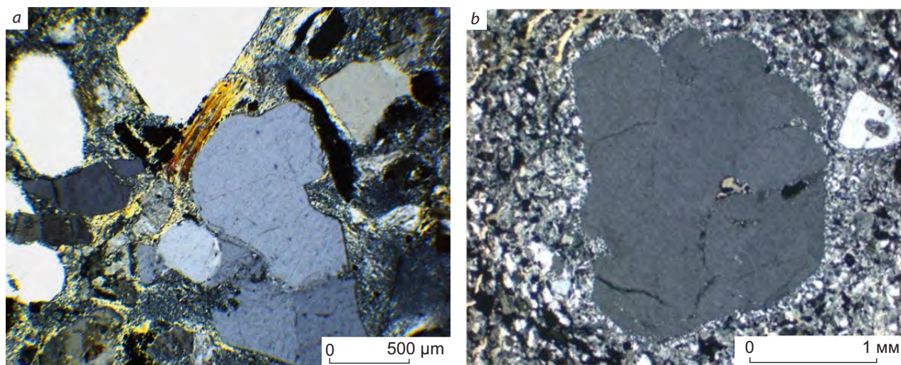
Рис. 5. Породы субвулканической фации:
