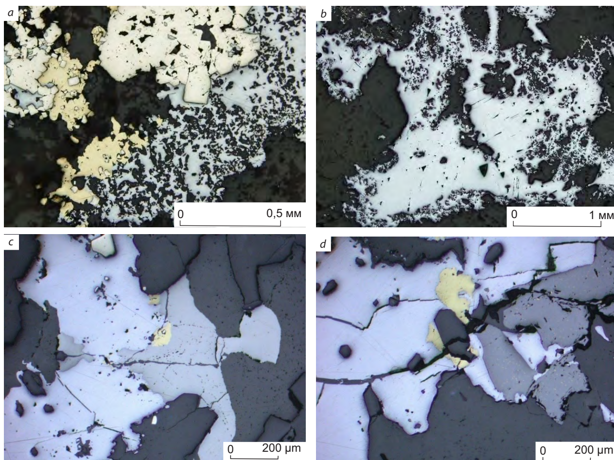
Рис. 7. Особенности свинцово-цинковых руд:
