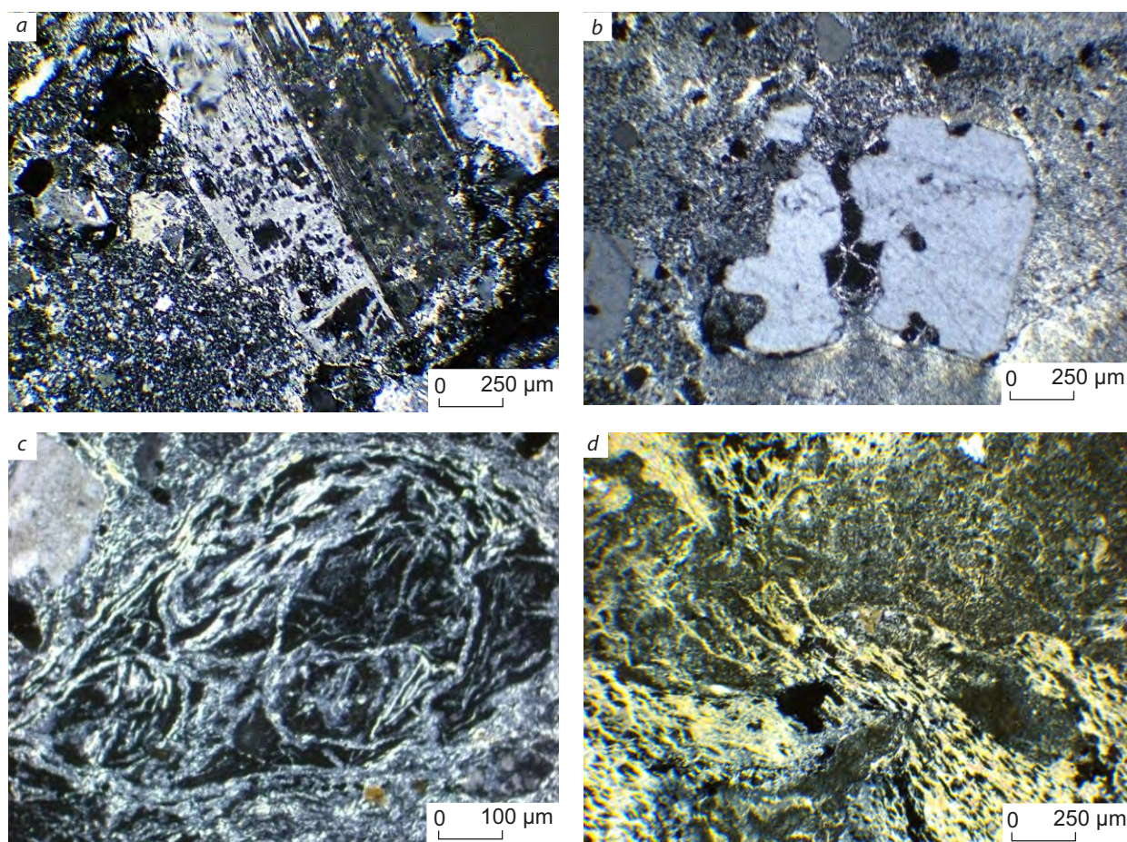
Рис. 4. Структурно-текстурные особенности игнимбритов:
