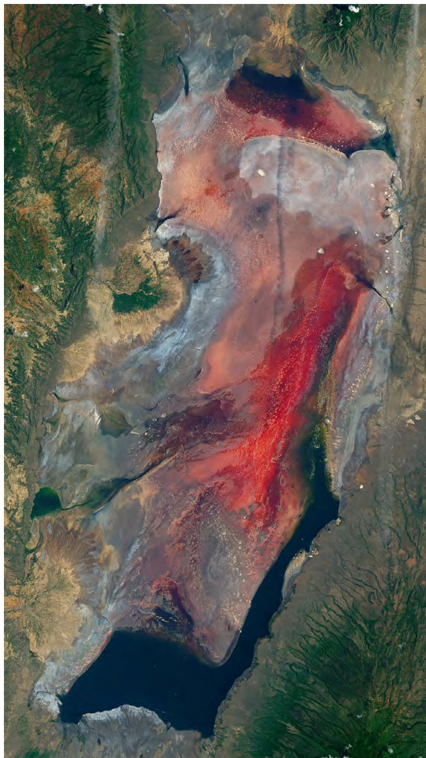
Рис. 2. Озеро Натрон и его структура, выраженная изменением цвета осадков дна
