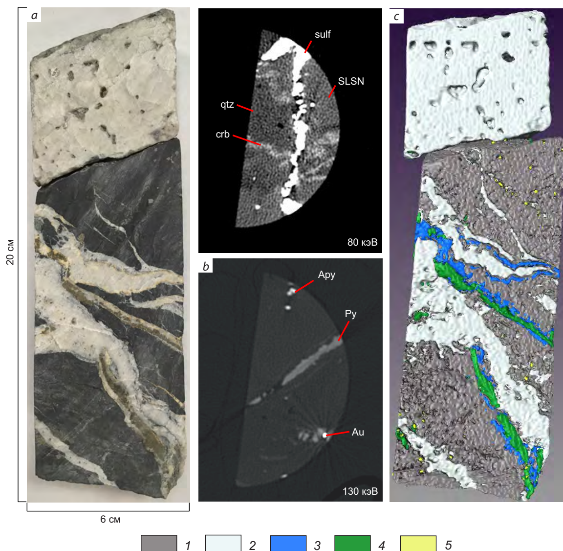
Рис. 3. Изучаемый образец керна и его стереологическая модель:
