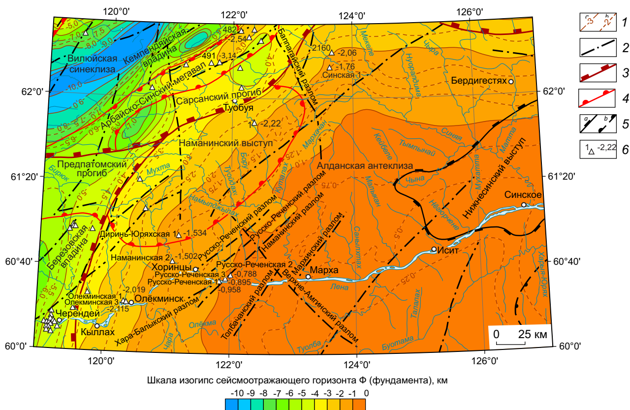
Рис. 5. Структуро-тектоническая схема фундамента (по материалам АО «Якутскгеофизика», НИГП АК «АЛРОСА» (ПАО)):
