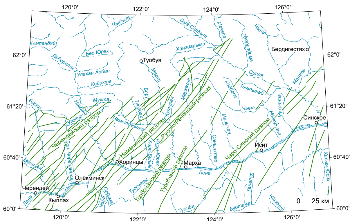
Рис. 1. Тектоническая схема Чаро-Синской площади (по данным АМС):
