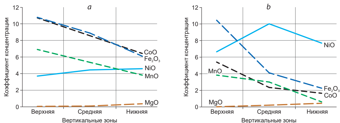
Рис. 3. Изменение коэффициента концентрации химических элементов в вертикальном профиле силикатно-никелевых руд месторождений Буруктаьское (а) и Сахаринское (б)
