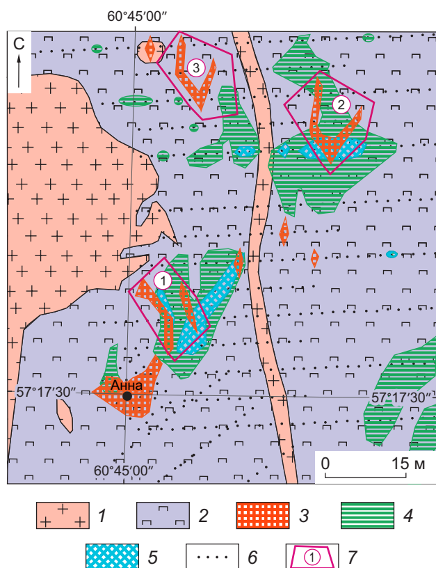
Рис. 4. Схема расположения ореолов привноса Au и Ni ( 0,6\% > \text{Ni} \geq 0,3\% ) рудного Первомайско-Верхотурского района:
