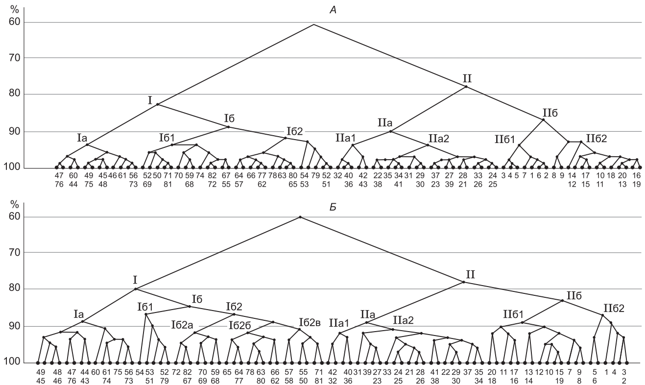
Рис. 1. Дендрограммы сходства локальных флор по спектрам:
