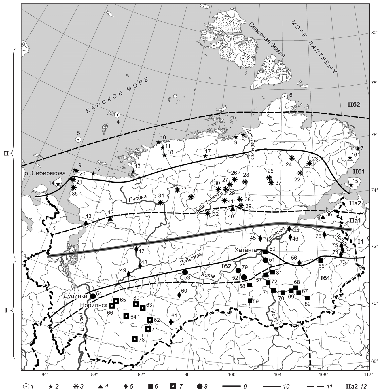
Рис. 2. Картографическое представление границ между кластерами и подкластерами с указанием типов и подтипов локальных флор (см. табл. 2).
