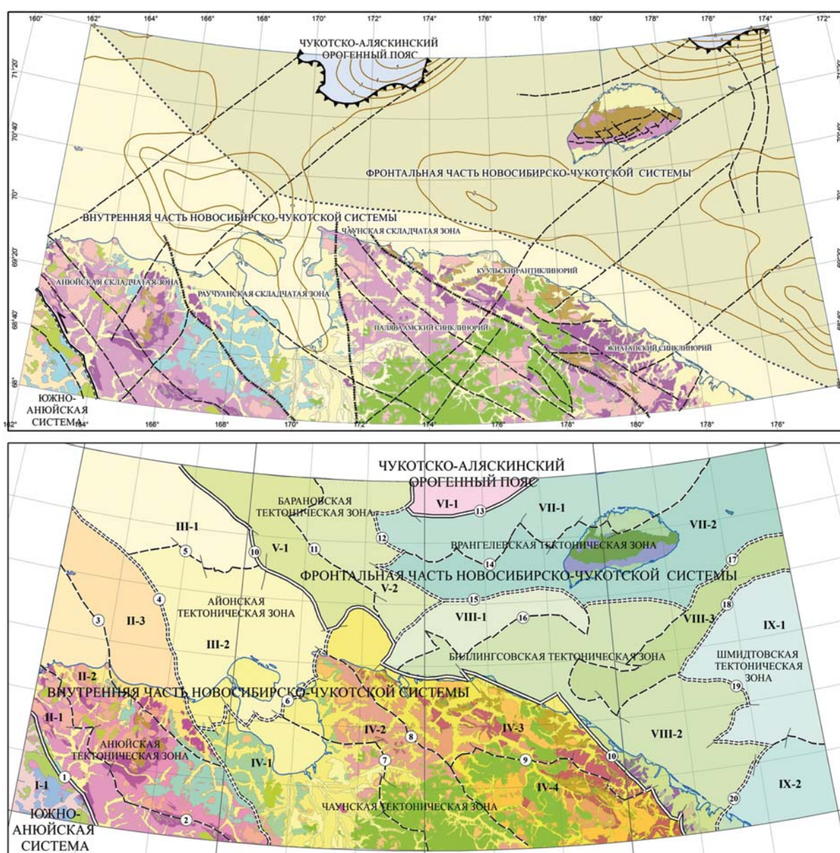
Рис. 1. Складчато-надвиговые системы и зоны на картах тектонического районирования по ретроспективным данным (ГГК-1000, сверху) и по геофизическим материалам (внизу) на площади листов R-58, 59, 60, 01
