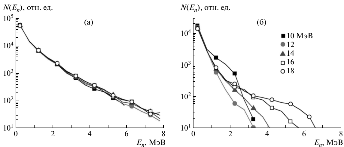
Рис. 2. Расчетный спектр нейтронов эффекта (а) и фона (б), выходящих из контейнера, при облучении тормозным излучением контейнера, заполненного железом, при различной энергии электронного пучка.
