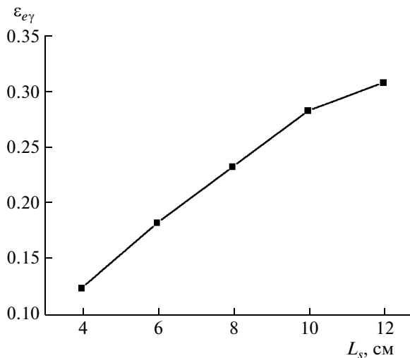
Рис. 9. Зависимость эффективности регистрации \gamma -квантов от толщины сцинтиллятора L_s при толщинах слоев 2 и 3: L_b = 0.5 см, L_p = 1.5 см.
