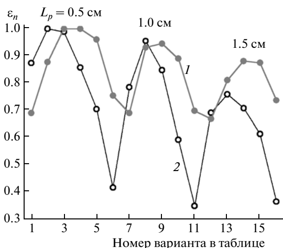
Рис. 7. Зависимость эффективности регистрации нейтронов от варианта конструкции детектора при разных фиксированных толщинах L_p слоя 2 (кривая 1 – мгновенные нейтроны эффекта, 2 – запаздывающие нейтроны).
