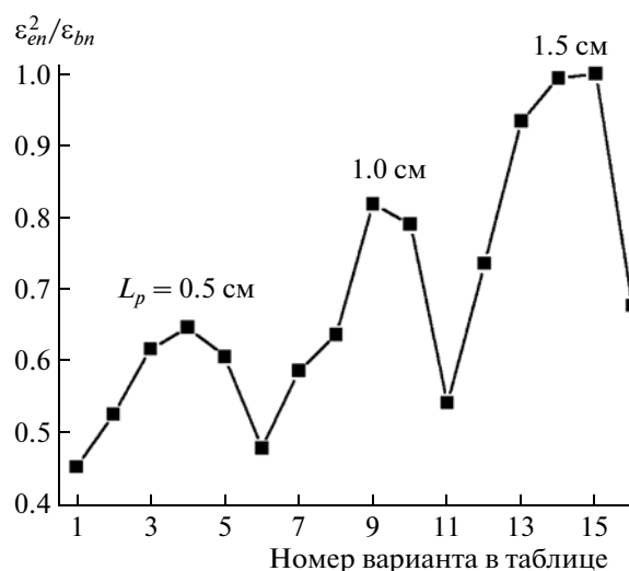
Рис. 8. Зависимость эффективности регистрации мгновенных нейтронов от варианта конструкции детектора при разных фиксированных толщинах L_p слоя 2.
