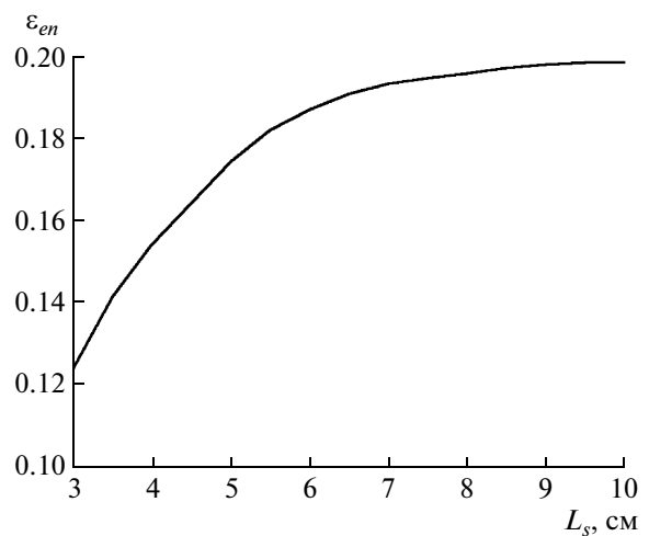
Рис. 6. Зависимость относительной эффективности регистрации нейтронов от толщины сцинтиллятора L_s (отражателя нейтронов).
