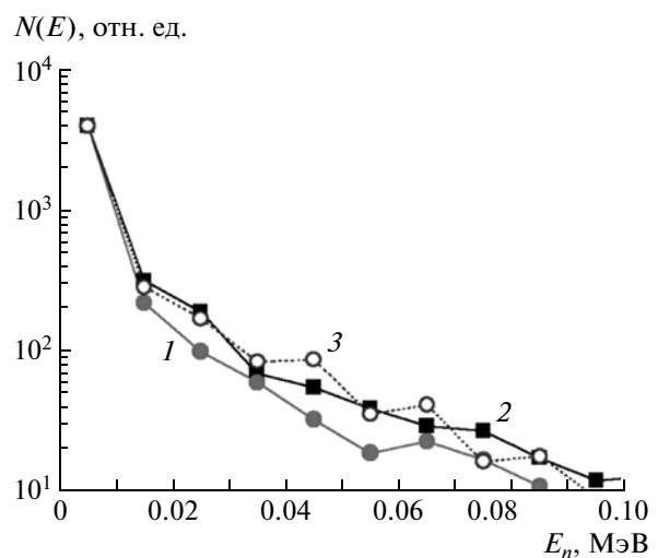
Рис. 11. Спектры нейтронов, приходящих на \gamma -детектор спустя 10 мкс после импульса тормозного излучения из контейнера, заполненного бумагой (1), алюминием (2), железом (3).
