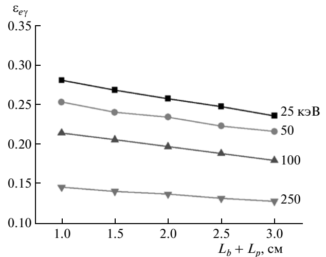
Рис. 10. Зависимость эффективности регистрации \gamma -квантов от суммарной толщины слоев L_b + L_p при различных энергетических порогах регистрации (значения у кривых).
