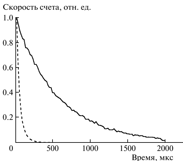
Рис. 12. Временная зависимость скорости счета мгновенных нейтронов (штриховая линия) и вторичных \gamma -квантов (сплошная линия) (данные нормированы на максимальное значение для каждого типа частиц).
