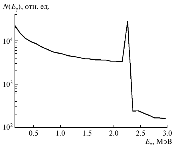
Рис. 3. Спектр вторичного \gamma -излучения из контейнера, заполненного водородосодержащим веществом (бумагой).
