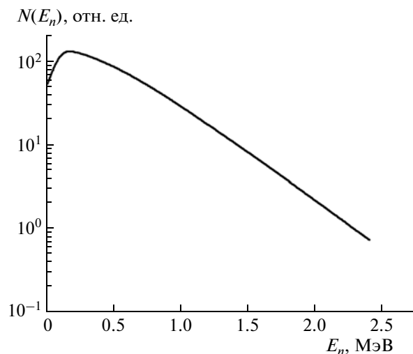
Рис. 4. Нормализованный спектр запаздывающих нейтронов деления.
