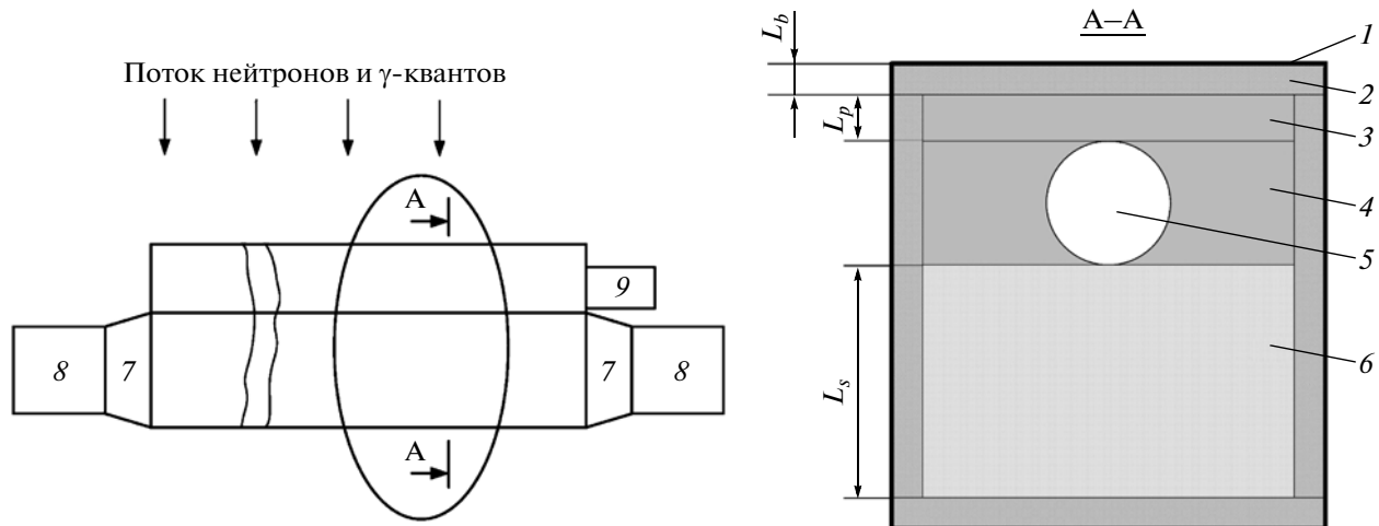
Рис. 5. Конструкция комбинированного детектора. 1 – слой кадмия, 2 – слой борированного полиэтилена, 3 – первый слой полиэтилена, 4 – второй слой полиэтилена, 5 – газонаполненный счетчик нейтронов, 6 – пластиковый сцинтиллятор, 7 – световоды, 8 – фотоэлектронный умножитель, 9 – предварительный усилитель.
