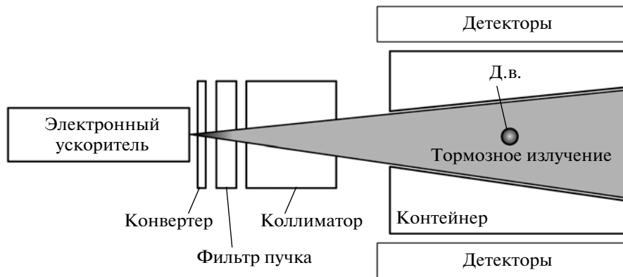
Рис. 1. Основные элементы установки для обнаружения д.в. фотоядерным методом.
