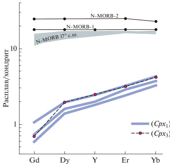
Рис. 8. Концентрации Gd, Dy, Y, Er и Yb в реакционном расплаве, рассчитанные по составу обогащенных Cpx_1 и Cpx_3 из наиболее высокотемпературной локальной ассоциации Op_{x3} + Spl_3 + Ol . Для сравнения показаны обобщенные составы N-MORB-1 и -2 (Sun, McDonough, 1989; Hofmann, 1988 соответственно). MORB 17° с.ш. — валовый состав базальтовых лав из НВП (см. рис. 1) в широтном интервале 17°06′–17°10′ с.ш. (В.Е. Бельтнев, неопубликованные данные). Концентрации элементов нормированы к хондриту C1 (Sun, McDonough, 1989).
