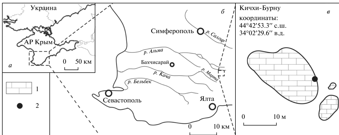
Рис. 1. Географическое положение и строение глыбы Кичхи-Бурну: а – Крымский полуостров, б – расположение местонахождения, в – схема олистолита Кичхи-Бурну. Обозначения: 1 – отложения олистолита Кичхи – Бурну; 2 – место находки трилобитов.
