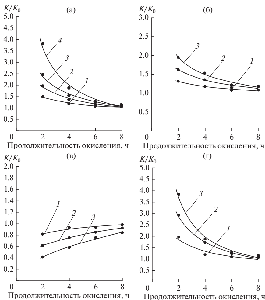
Рис. 1. Зависимость эффекта процесса окисления модифицированного гудрона от продолжительности окисления: а) тяжелая нефтяная пиролизная смола: 1, 2, 3, 4 – окисленный битум из нефтяного гудрона, содержащего 0.5, 1.5, 3.0 и 5.4 мас. % модификатора соответственно; б) смола пиролиза горючих сланцев Туровского месторождения: 1, 2, 3 – окисление нефтяного гудрона, содержащего 1.5, 3.0 и 5.0 мас. % модификатора соответственно; в) смола пиролиза бурых углей Лельчицкого месторождения: 1, 2, 3 – окисление нефтяного гудрона, содержащего 1.5, 3.0 и 5.0 мас. % модификатора соответственно; г) алмазосодержащая шихта: 1, 2, 3 – окисление нефтяного гудрона, содержащего 0.06, 0.15 и 0.22 мас. % модификатора соответственно.
