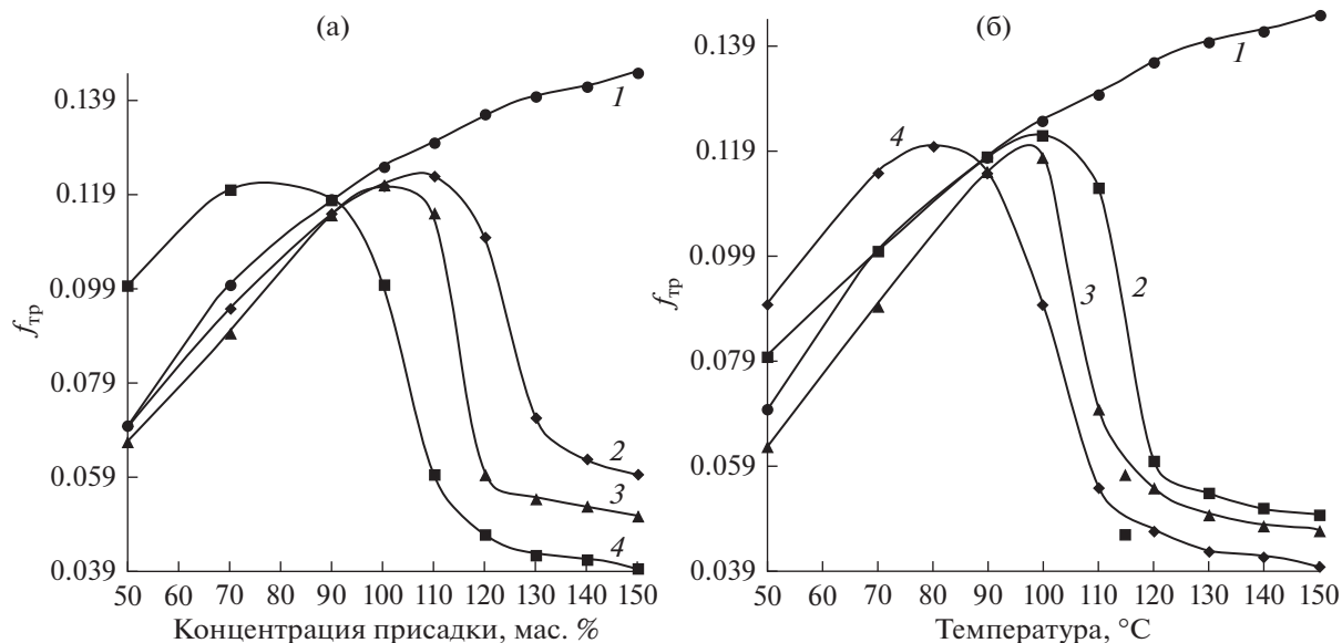
Рис. 5. Зависимость коэффициента трения от температуры для наночастиц \text{MoS}_3 , полученных из [\text{CH}_3(\text{C}_8\text{H}_{17})_3\text{N}]_2\text{MoS}_4 (а) и [\text{CH}_3(\text{C}_8\text{H}_{17})_3\text{N}]_2\text{MoS}_4 (б), при различной концентрации молибдена: 1 – чистое вазелиновое масло, 2 – концентрация \text{MoS}_3 100 ppm, 3 – концентрация \text{MoS}_3 250 ppm, 4 – концентрация \text{MoS}_3 500 ppm.
