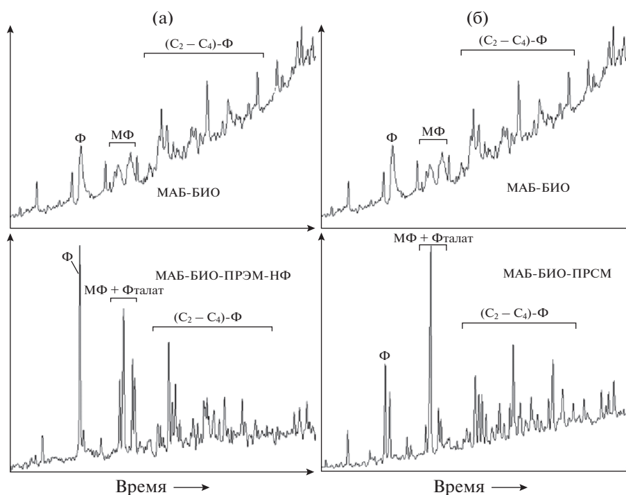
Рис. 4. Изменение молекулярно-массового распределения фенантронов ( m/z 178 + 192 + 206 + 220 + 234) после разрушения эфирных (а) и сульфидных (б) мостиков. Ф – фенантрен, МФ, ( C_2-C_4 ) – области элюирования гомологов фенантрена.
