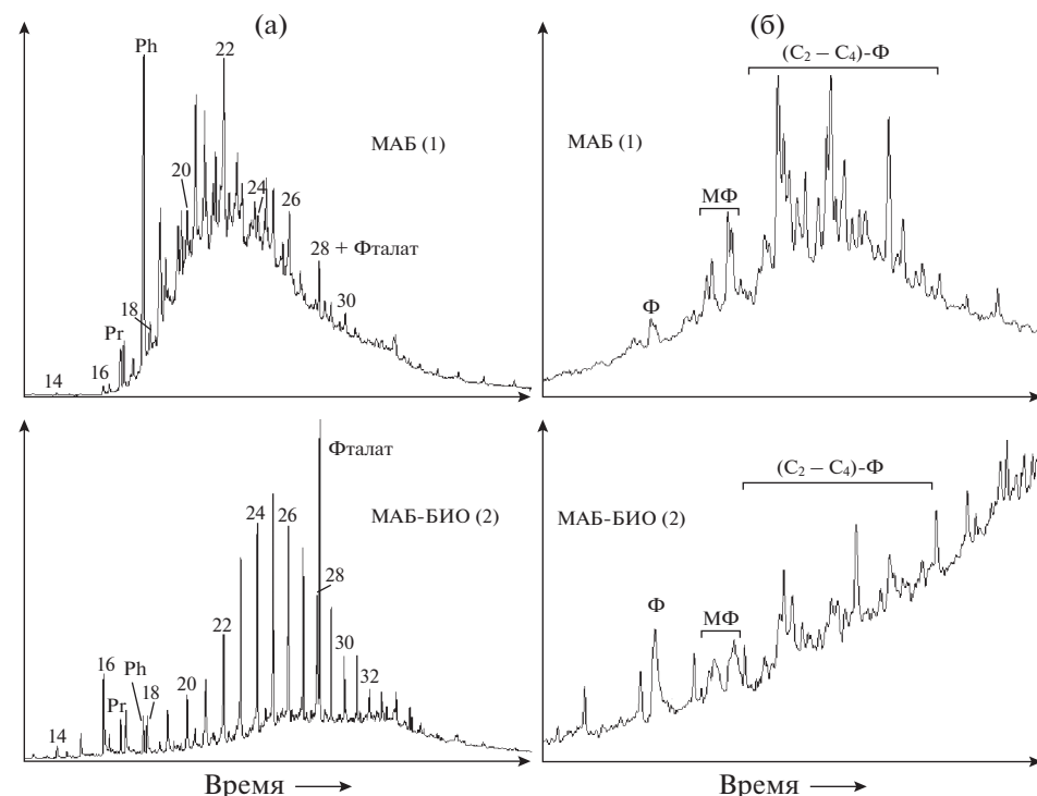
Рис. 1. Масс-хроматограммы алканов (а, m/z 57) и фенантронов (б, m/z 178 + 192 + 206 + 220 + 234) в маслах исходной (1) и биоградирированной (2) нефти. Цифры соответствуют числу атомов углерода в молекуле n -алканов. Ф — фенантрен, МФ — метилфенантроны, (C_2-C_4) -Ф — области элюирования гомологов фенантрена.
