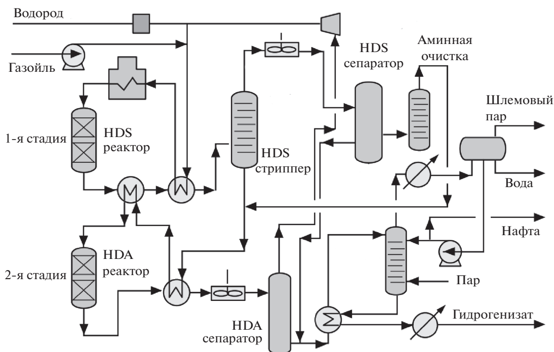
Рис. 3. Схема процесса "TopsøeUDHDS". Адаптировано из [58].
