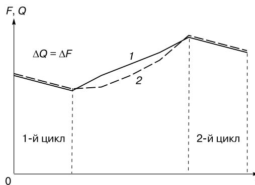
Рис. 4. Изменение во времени T значений сил сопротивления мерзлого грунта деформации F (1) и сил сопротивления талого грунта сжатию Q (2) для двух циклов пучения.
