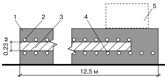
Рис. 2. Продольный разрез фундаментного модуля.
