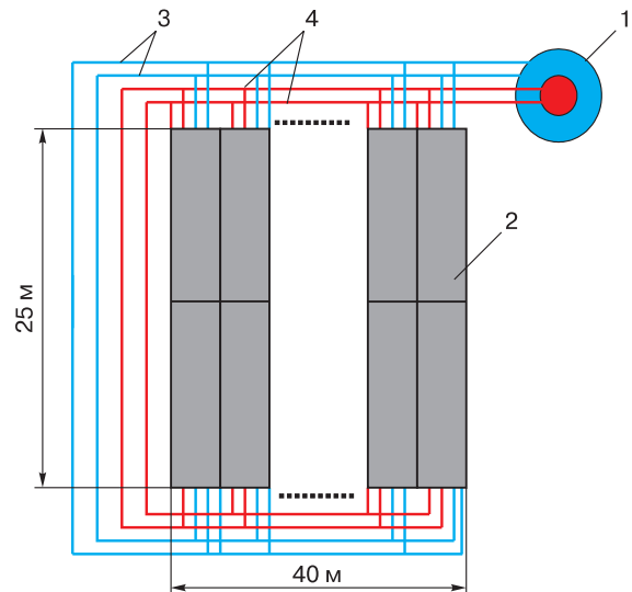
Рис. 3. Схема подключения фундаментных модулей к тепловому насосу.
