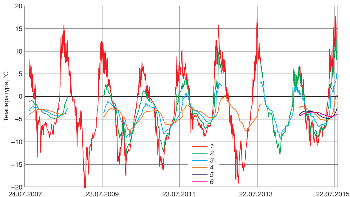
Рис. 7. Динамика температуры в скважине SB 03 на поверхности морской лайды в зоне современной морской аккумуляции на разных глубинах:
