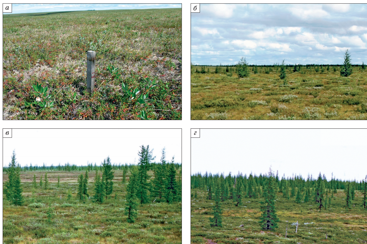
Рис. 8. Изменение растительного покрова на Южном Уренгее при потеплении климата.
