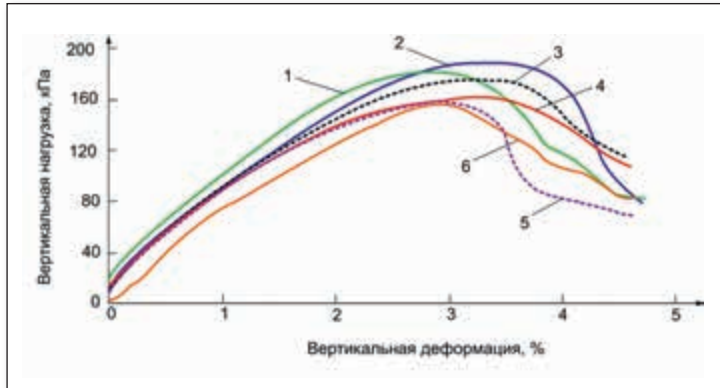
Рис. 6. Зависимость вертикальной деформации от вертикальной нагрузки (напряжения) при различном количестве циклов замораживания-оттаивания [42]: 1 — два цикла; 2 — ноль циклов (незамороженный грунт); 3 — пять циклов; 4 — одиннадцать циклов; 5 — двадцать один цикл; 6 — тридцать один цикл
