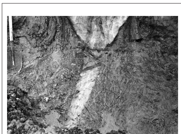
Рис. 11. Узкий хвост в нижней части широкой жилы с деформациями вмещающих пород на контакте в нижнем фрагменте толщи поймы устьевой части реки Тамбей. Верхняя часть хвоста жилы находится на меженном уровне реки (фото Ю.К. Васильчука)
