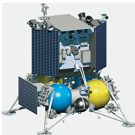
Общий вид АМС “Луна-25” (проект “Луна-Глоб”). Рисунок “НПО им. С.А. Лавочкина”
