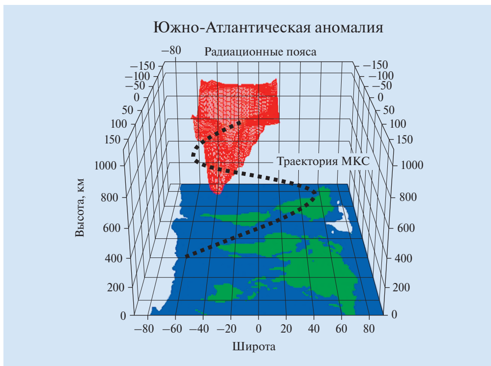
Радиационные пояса Земли над Южной Атлантикой. Именно здесь, на высоте около 400 км, МКС пересекает область повышенного уровня радиации
