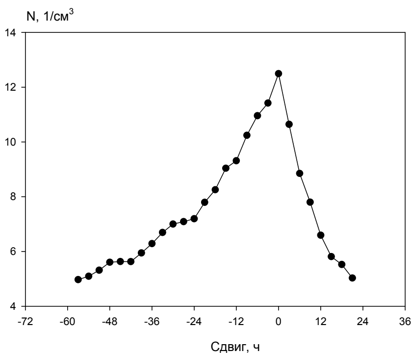
Рис. 5. Распределение средних значений плотности СВ в окрестности реперных точек, отобранных по критерию K_p(3 \text{ ч}) > 4 , таких, что расстояние до предыдущего значения K_p(3 \text{ ч}) > 4 составляет не менее трех суток
