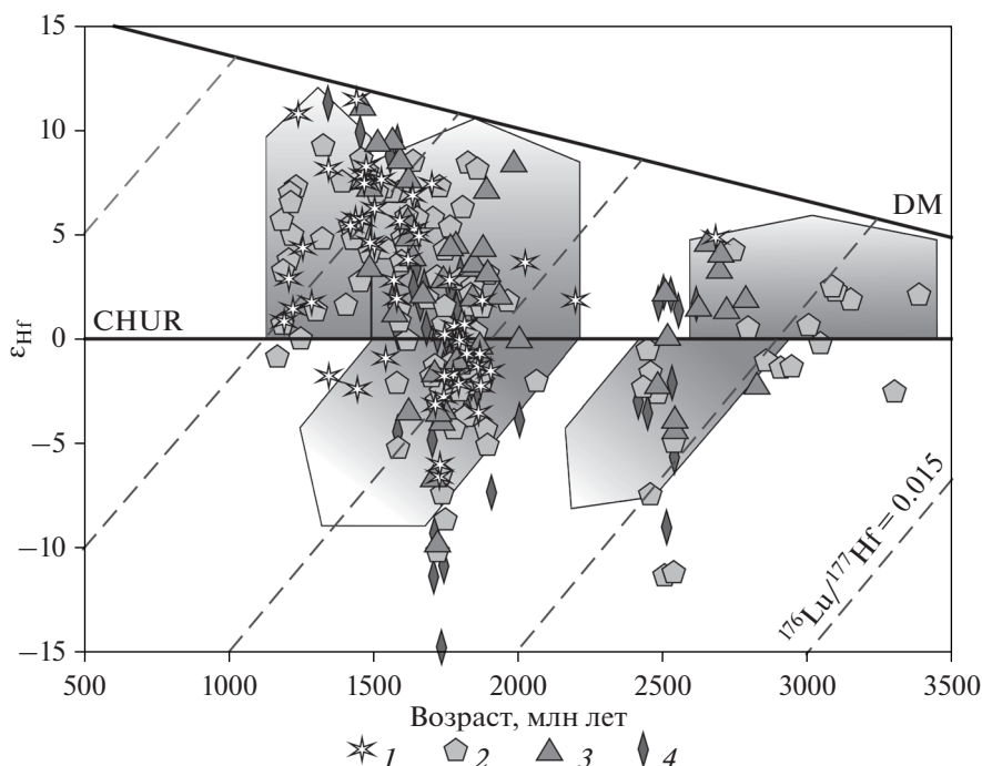
Рис. 7. Диаграмма зависимости \epsilon_{\text{Hf}} –Возраст (млн лет) для конкордатных детритовых цирконов, отражающая эволюцию докембрийской континентальной коры Актау-Моинтинского массива в докембрии. 1–4 – фигуративные точки цирконов из проб: 1 – Б-15118, 2 – Б-15102 и Б-15103, 3 – Б-15108 4 – АМ-1711
