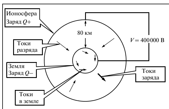
Рис. 1. Модель Земли и ионосферы в виде шарового конденсатора.
