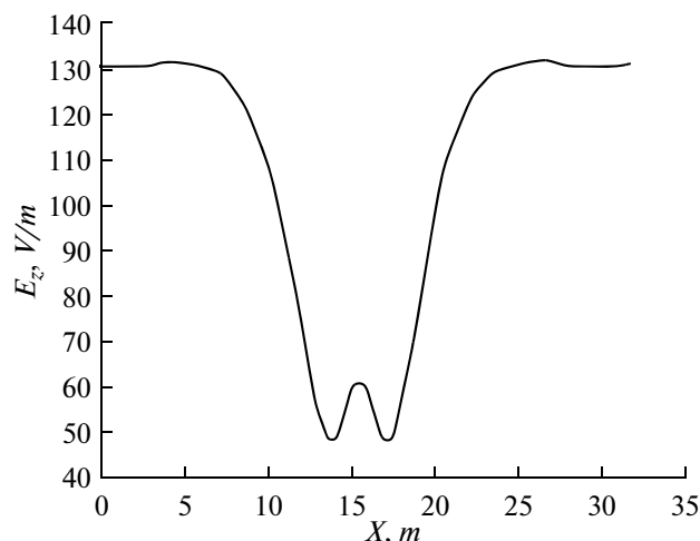
Рис. 4. Зависимость напряженности вертикальной компоненты электрического поля с повышенной проводимостью.
