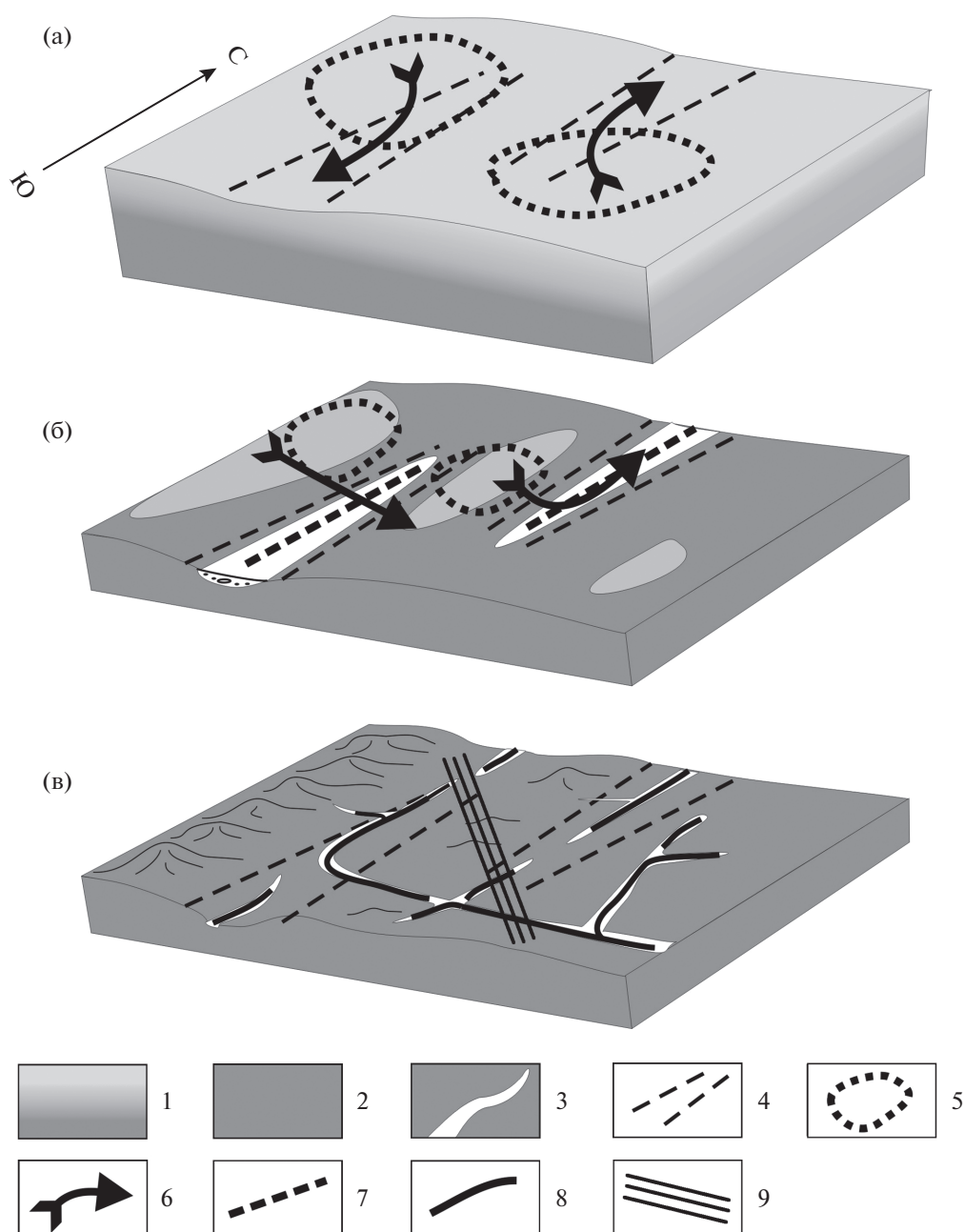
Фиг. 5. Эволюционная трансформация рудно-россыпной системы Вагранского узла. Этапы: а – позднемезозойский–раннекайнозойский этап пенеplanation; б – начало тектонической активизации (олигоцен–плиоцен); в – формирование современного рельефа (плейстоцен–голоцен). 1 – коры выветривания; 2 – метаморфизованные отложения складчатого комплекса; 3 – аллювиальные отложения; 4 – эрозионно-структурные депрессии (ЭСД); 5 – предполагаемые выходы россыпеобразующих коренных источников; 6 – направления переноса обломочного материала; 7 – водотоки в пределах ЭСД; 8 – современные водотоки; 9 – предполагаемая зона серебряно-золотой минерализации типа V на современном эрозионном уровне.
