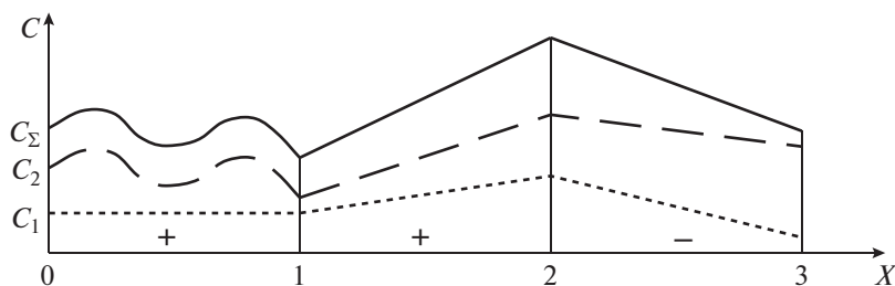
Фиг. 12. Влияние распределения раннего алунита с низкой МДК и позднего с высокой МДК на корреляцию SO 3 ~МДК. По вертикальной оси отложены содержания алунита (С): раннего (С 1 , пунктирная линия), позднего (С 2 , прерывистая линия), общее (С Σ , сплошная линия). Горизонтальная ось отражает условное расстояние (Х) от начала разведочной выработки. Знаки “+” и “-” показывают знак корреляции на отрезках.
