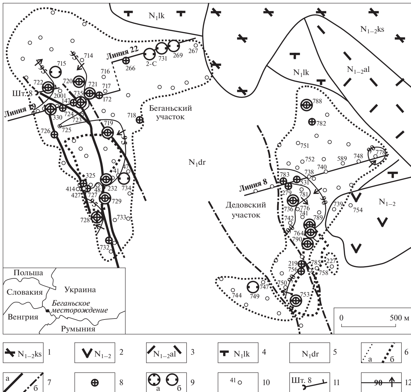
Фиг. 1. Геологическая схема Беганьского месторождения (составил А.З. Вдовец с использованием разведочных материалов Ю.В. Сабова). 1 – глины, пески, туффиты кошелевской свиты; 2 – андезито-базальты; 3 – глины, туфопесчаники и др. алмашской свиты (сармат); 4 – алевролиты, туффиты и др. луковской свиты (нижний сармат); 5 – липаритовые туфы доробратовской свиты (нижний сармат); 6 – контуры: а – алунитовых кварцитов, б – монокварцитов; 7 – разрывные нарушения: а – вмещающие барит-полиметаллические руды, б – безрудные; 8–9 – скважины со значимой корреляцией: 8 – SO 3 ~МДК (положительной), 9 – SO 3 ~СКН (а – положительной, б – отрицательной); 10 – скважины, в которых значимая корреляция не установлена; номера указаны только у скважин, по которым имелись результаты определения калия и натрия; 11 – штольня с рассечкой и ее номер; 12 – изолинии средних значений МДК по скважинам, стрелка показывает направление возрастания МДК.
