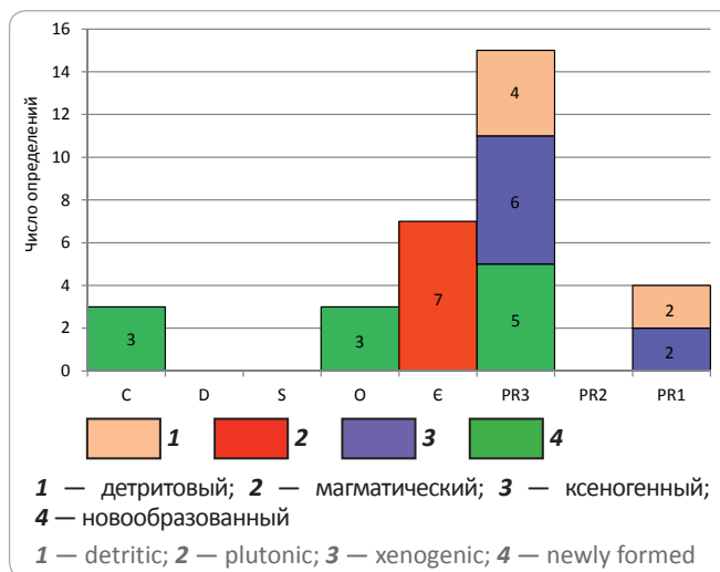
Рис. 3. Распределение датировок цирконов разного генезиса из метаморфических пород южной зоны (зона II) Fig. 3. Dating distribution for zircon of different genesis from metamorphic rocks in the southern zone (Zone II)
