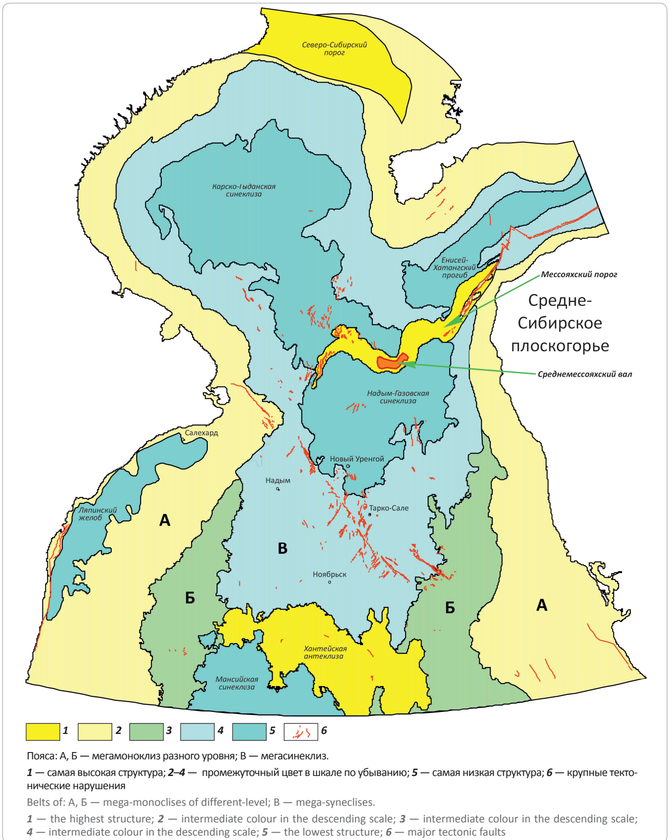
Рис. 1. Тектоническая карта мезо-кайнозойского ортоплатформенного чехла Западной Сибири (Бочкарев В.С. и др., 2001) Fig. 1. Tectonic map of Mesozoic-Cenozoic orthoplatform cover, West Siberia (Bochkarev V.S. et al., 2001)
