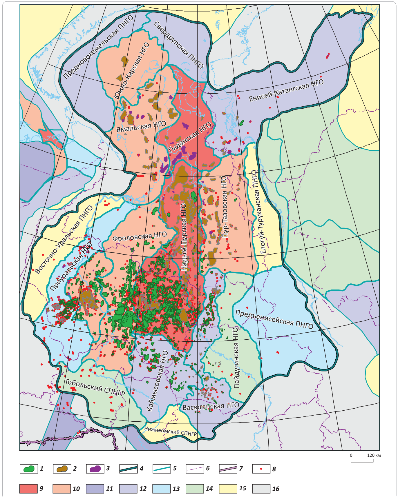
Рис. 4. Схема нефтегазоносности Западно-Сибирской НПП Fig. 4. Scheme oil and gas occurrence over the West Siberian Petroleum Province
