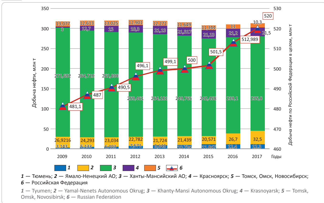
Рис. 1. Сравнительная динамика добычи нефти в Российской Федерации и Западно-Сибирской НГП Fig. 1. Comparative oil production history of Russian Federation and West Siberian Petroleum Province
