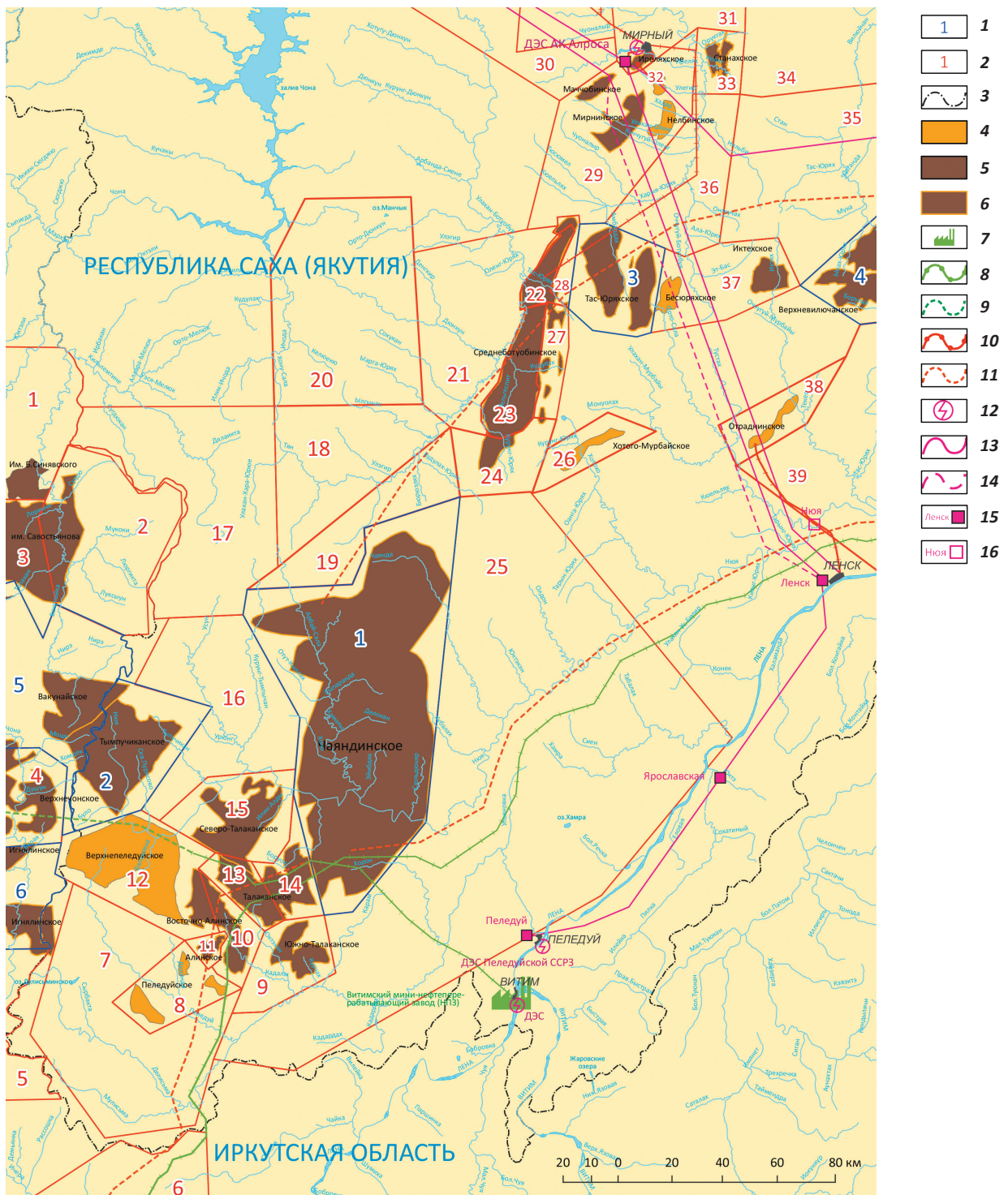
Рис. 1. Обзорная карта района работ Чаюдинского НГКМ Fig. 1. Location map of study area showing the Chayandinsky oil and gas condensate field
