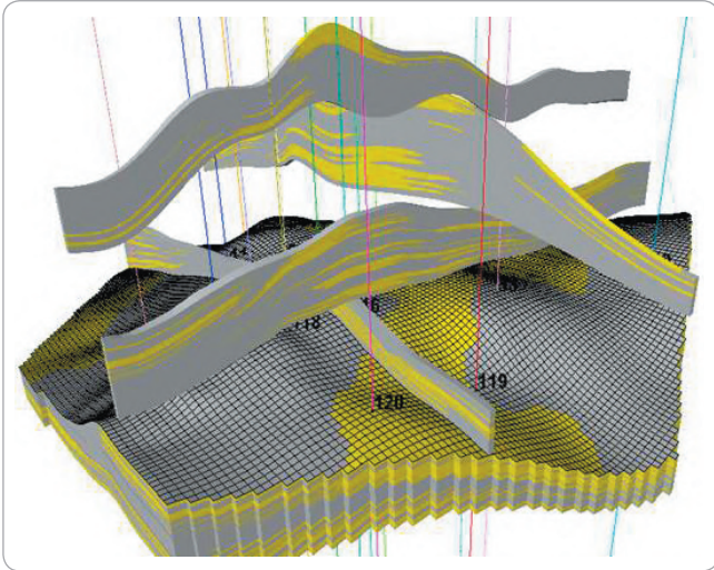
Рис. 11. Геологическая модель месторождения левобережной части Астраханского ГКМ (фрагмент куба литологии) Fig. 11. Geological model of the field in the left-bank part of the Astrakhansky gas condensate field (fragment of lithology cube)
