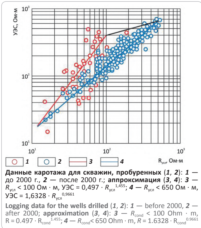
Рис. 6. Зависимость УЭС от условного сопротивления, определенного по данным БК-3 (Астраханское ГКМ) Fig. 6. Resistivity as a function of conventional resistivity determined from LL-3 data (Astrakhansky gas condensate field)
