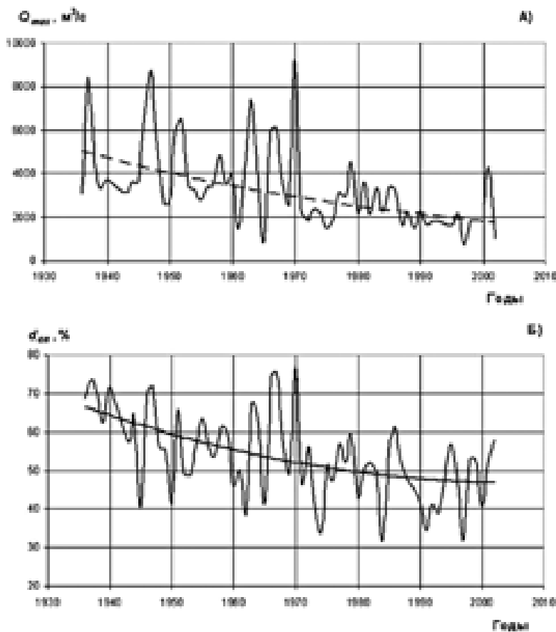
Рис. 9. Изменение максимальных расходов воды, м 3 /с (а) р. Ока (г. Калуга) и доли половодья в годовом стоке, % (б) за период 1935–2005 гг.
