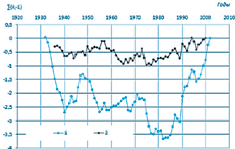
Рис. 5. Разностная интегральная кривая среднегодовых расходов воды р. Уфы (г. Красноуфимск) (1) и сумм годовых осадков (2).
