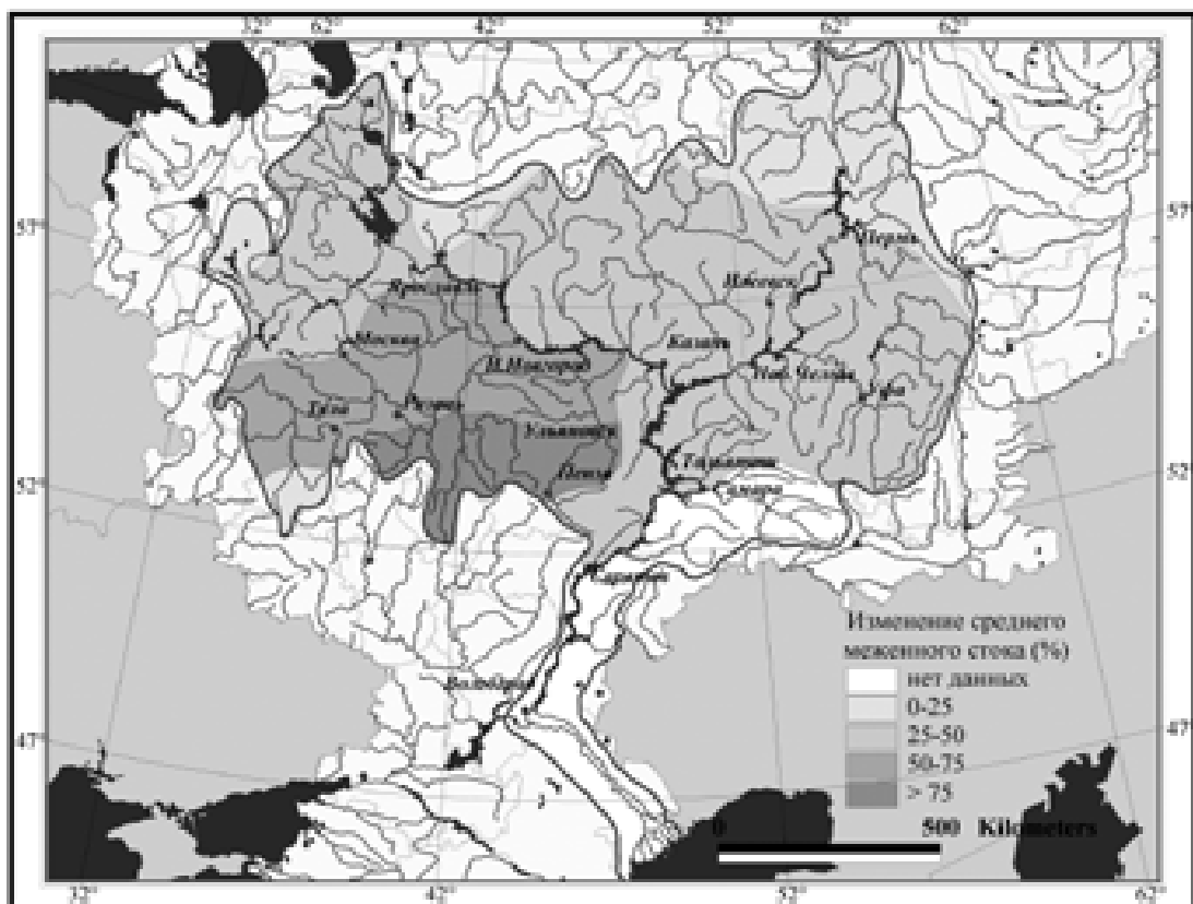
Рис. 10. Изменение среднего меженного (подземного) стока (%) за 1970–2005 гг. по сравнению с периодом 1935–1969 гг.
