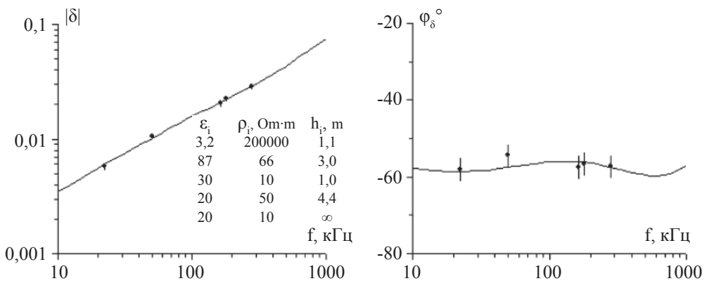
Рис. 1. Результаты интерпретации модуля и фазы импеданса, измеренных на 5 частотах ОНЧ-НЧ-диапазонов в пункте наблюдений № 4 опорного профиля в заливе Провал. Сплошные линии – зависимости импеданса для восстановленного разреза, точки – экспериментальные значения импеданса
