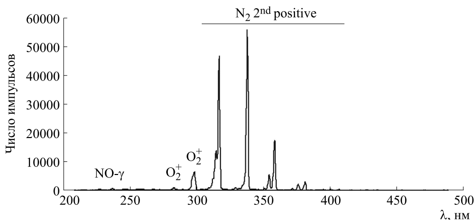
Рис. 1. Спектр излучения прямого пьезоразряда в воздухе при атмосферном давлении в диапазоне 200–500 нм.
