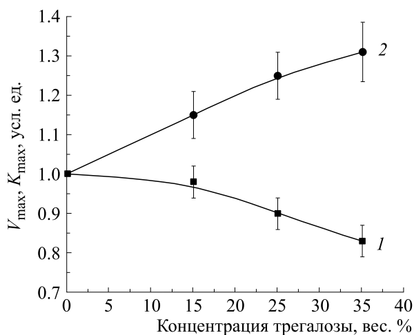
Рис. 4. Зависимости максимальной скорости гидролиза АТФ ( V_{\max} ) и кажущейся константы Михаэлиса ( K_m ) реакции от концентрации трегалозы. За единицу принята максимальная скорость, равная 11,2 \text{ мкмоль} \cdot \text{мин}^{-1} \text{ мг}^{-1} (1), и константа Михаэлиса, равная 1,03 \text{ мМ} (2).
