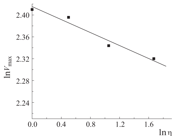
Рис. 5. Зависимость скорости гидролиза АТФ от вязкости реакционной среды в логарифмических координатах.
