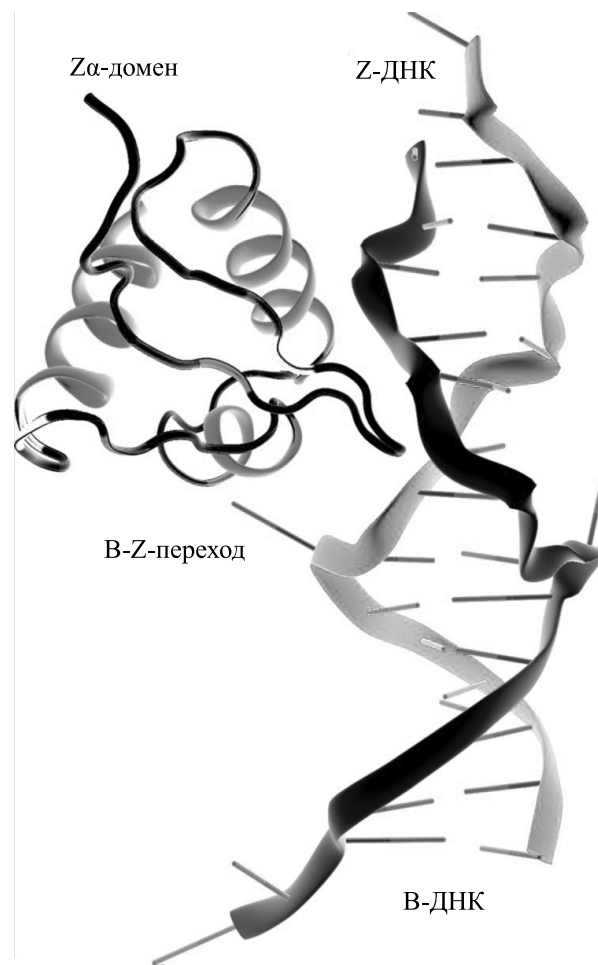
Рис. 4. Взаимодействие Z\alpha -домена Z-ДНК связывающегося белка с Z-ДНК на примере белка ADAR1 [73].
