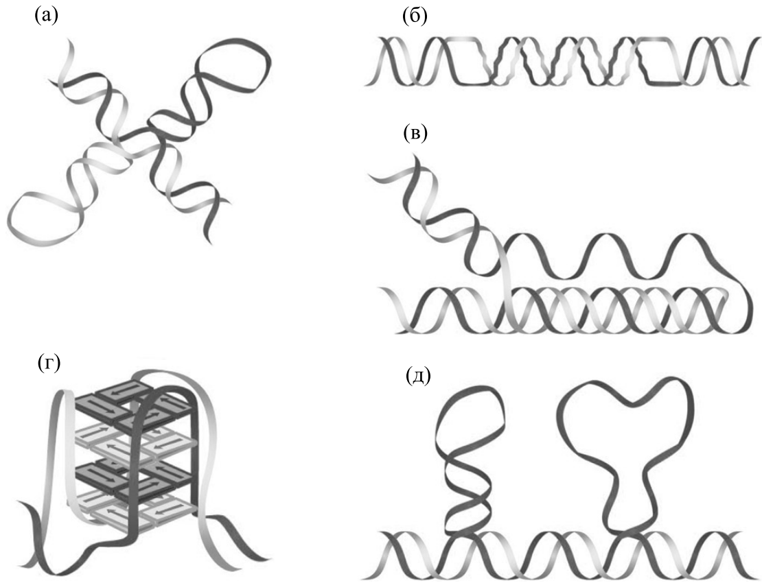
Рис. 1. Неканонические формы спирали ДНК: (а) – крестовидная форма, (б) – Z-ДНК, (в) – H-ДНК (тройная спираль), (г) – G-ДНК (квадруплекс), (д) – шпильки и петли ДНК [2].
