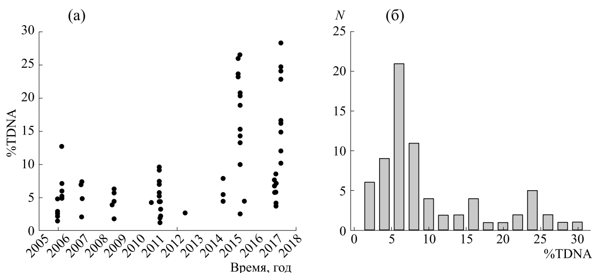
Рис. 1. Распределение значений %TDNA лейкоцитов крови интактных мышей из использованного массива данных по датам экспериментов (а) и по наблюдаемым величинам (б).
