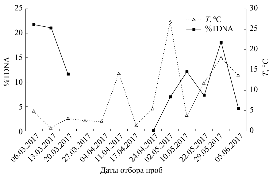
Рис. 6. Изменения %TDNA клеток АКЭ и среднесуточной температуры воздуха в дни отбора асцита. Уровень повреждений ДНК представлен как разность средних значений %TDNA облученных и необлученных клеток АКЭ.
