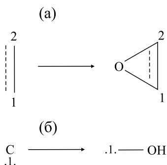
Рис. 1. Фрагменты используемых реакций биотрансформации: (а) – реакция эпексидирования, (б) – реакция С-гидроксилирования.
