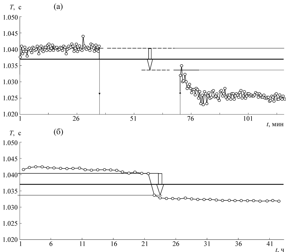
Рис. 12. (а) – Фрагмент рис. 11 в окрестности периода 1,037 с при большем увеличении по вертикали. В узкой окрестности этого периода УСУП расположена симметричная область ( \pm 0,3\% ) запрещенных значений периода тестируемого RC-генератора периодических колебаний. (б) – Результат аналогичного опыта, выполненного при другой настройке RC-генератора. Симметричная область запрещенных значений периода УСУП, обнаруженная в этом опыте, совпадает с областью запрещенных значений периода УСУП в опыте, представленном на рис. 12а.
