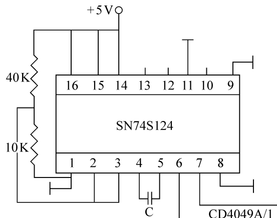
Рис. 4. Ядро RC-генератора периодических колебаний. Для того чтобы начальный период генератора попадал в область околосекундных периодов, емкость C выбирали из широкой окрестности 1000 мкФ. Сопряжение с компьютером, как на предыдущих схемах.
