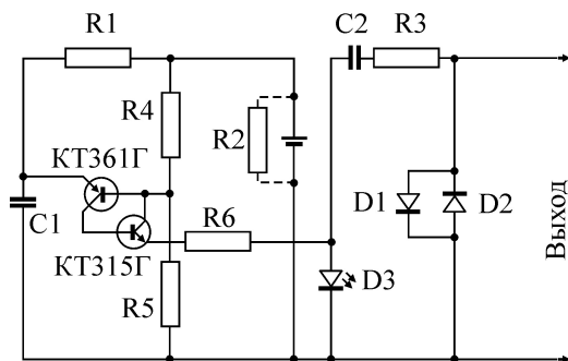
Рис. 3. Принципиальная схема релаксационного генератора на тиристоре, реализованного посредством транзисторов КТ315Г и КТ361Г. Светодиод D3 – индикатор/визуализатор импульсов.
