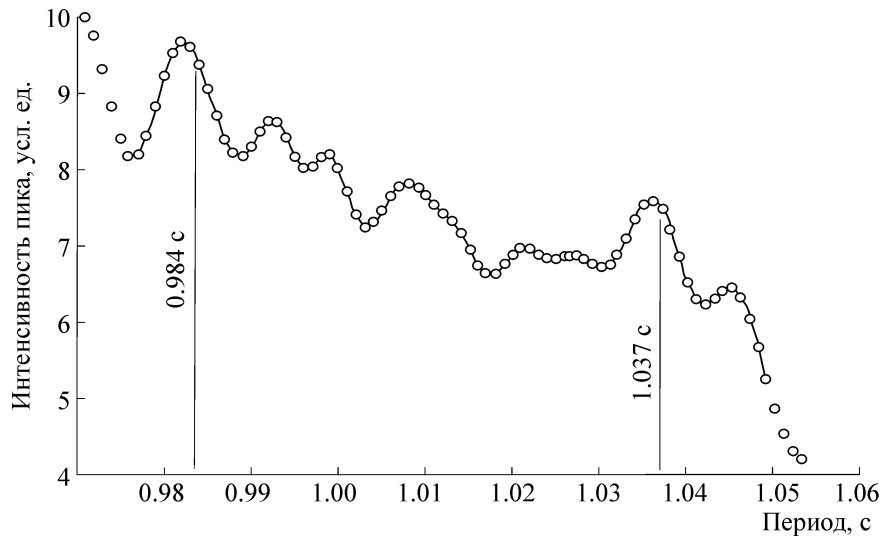
Рис. 13. Соседние уровни УСУП T_{-20;0} = 1,037 с и T_{-15;8} = 0,984 с найдены в ходе сканирования посредством 12-разрядного цифро-аналогового преобразователя периода хорошо термостабилизированного генератора периодических колебаний. Экспериментальный ряд чисел сглажен 12-кратным применением алгоритма Y_i^{n+1} = (Y_{i-1}^n + 2Y_i^n + Y_{i+1}^n)/4 .
