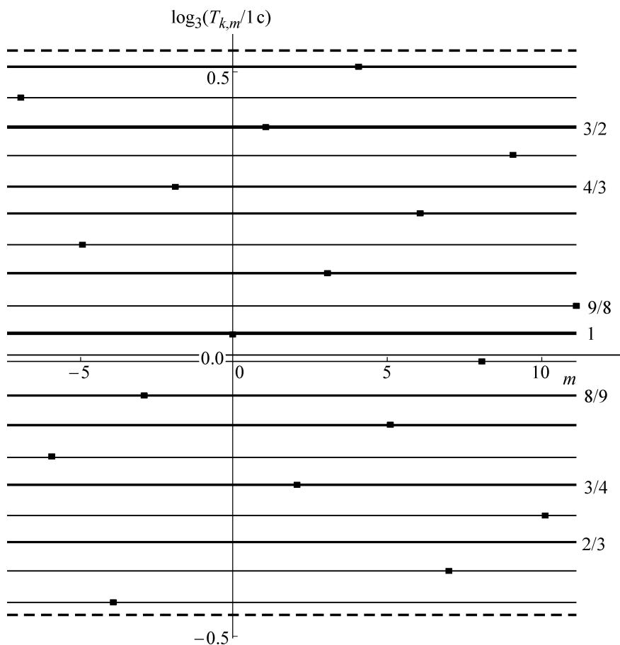
Рис. 15. Страта УСУП в окрестности периода T_{-20;0} = 1,037 с. Две наиболее жирные линии отвечают периодам с m = 0 и 1 , отмеченным еще в пионерской работе [1]. Верхняя и нижняя границы страты помечены горизонтальными штриховыми линиями, это вспомогательные линии рисунка. Выше и ниже этой страты находятся страты с точно таким же распределением резонансов по отношению к соответствующим центральным периодам страт, т.е. по отношению к периодам ..., 9 \cdot 1,037 с, 3 \cdot 1,037 с, а также 1,037/3 с, 1,037/9 с, ... , что в итоге дает полное представление об УСУП.
