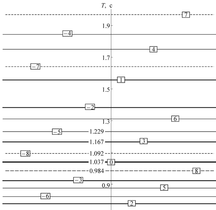
Рис. 14. Фрагмент спектра периодов УСУП в окрестности уровня T_{-19;1} = 1,555 с (ср. с рис. 5–12). Вдоль вертикальной оси отложены значения периодов УСУП, горизонтальная ось играет вспомогательную роль: периоды УСУП изображены как горизонтальные уровни, толщина которых качественно отражает значимость периода, вероятность его наблюдения. Цифры в прямоугольниках показывают значения параметра m для каждого из уровней; вероятность обнаружения уровня T_{k,m} (толщина линии) заметно падает с ростом абсолютной величины m .
