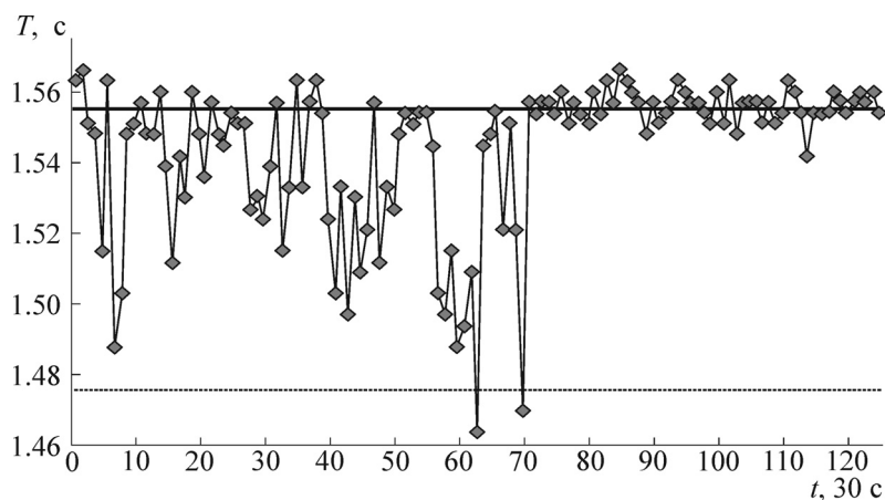
Рис. 8. Выбросы (резко возросшие флуктуации) в момент пересечения периодом RC-генератора окрестности дискретного уровня УСУП T_{-19;1} = 1,555 с. В течение 30-секундного измерения эти выбросы могут возникать из-за смешивания неизменных дискретных значений периода T_{-19;1} \approx 1,555 с и результатов произошедших за эти 30 с кратковременных переходов на другие дискретные уровни УСУП. При этом среднечасовое значение периода наблюдается тоже как некий выброс с уровня T_{-19;1} (рис. 7 и 9).
