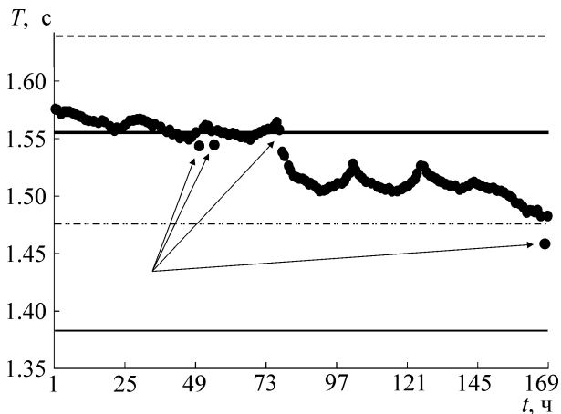
Рис. 7. Серия аномальных выбросов в результатах среднечасовых измерений периода RC-генератора. Моменты возникновения аномалий коррелируют с моментами совпадения дрейфующего периода RC-генератора с уровнями УСУП.
