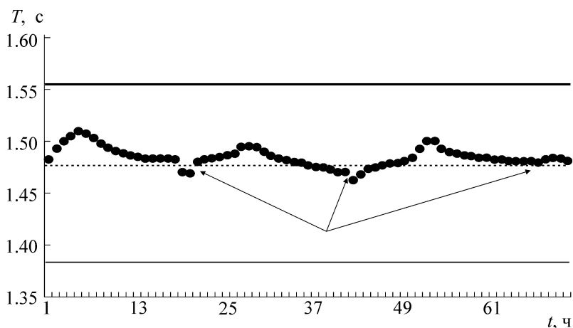
Рис. 9. Продолжение опыта, представленного на рис. 7. Зона аномальных значений периода (выбросов) располагается теперь в окрестности уровня T_{-14;9} = 1,476 с.
