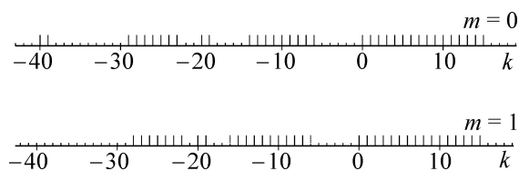
Рис. 1. Фрагмент исследованного диапазона периодов, где помечены обнаруженные периоды T_{k,m} = P_0 \cdot 3^{k/2^m} , входящие в УСУП. Масштаб логарифмический. Астрономические, гео- и биологические периоды T_{k,m} , занимающие диапазон k = 0 \div 15 , описаны в работе [1], биофизические периоды T_{k,m} , найденные в окрестности k = -10 и k = -25 , представлены в работах [2–5], технические периоды T_{k,m} , обнаруженные в сверхвысокочастотной области в окрестности k = -40 , см. в работах [6–8].
