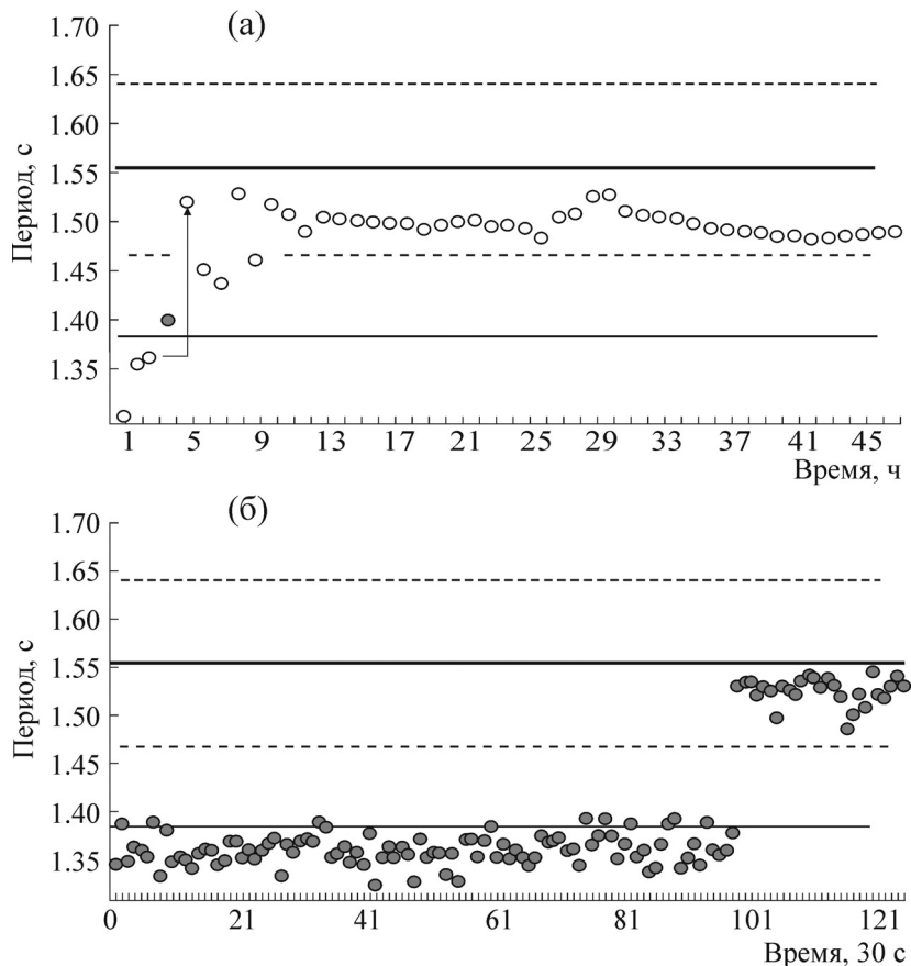
Рис. 6. Скачок значений периода RC-генератора из окрестности уровня T_{-21;-2} = 1,383 с в окрестность уровня T_{-19;1} = 1,555 с в момент дрейфа периода RC-генератора периодических колебаний через окрестность уровня УСУП T_{-21;-2} . Вверху график среднечасовых значений в течение двух суток, внизу – полуминутных в течение часа.
