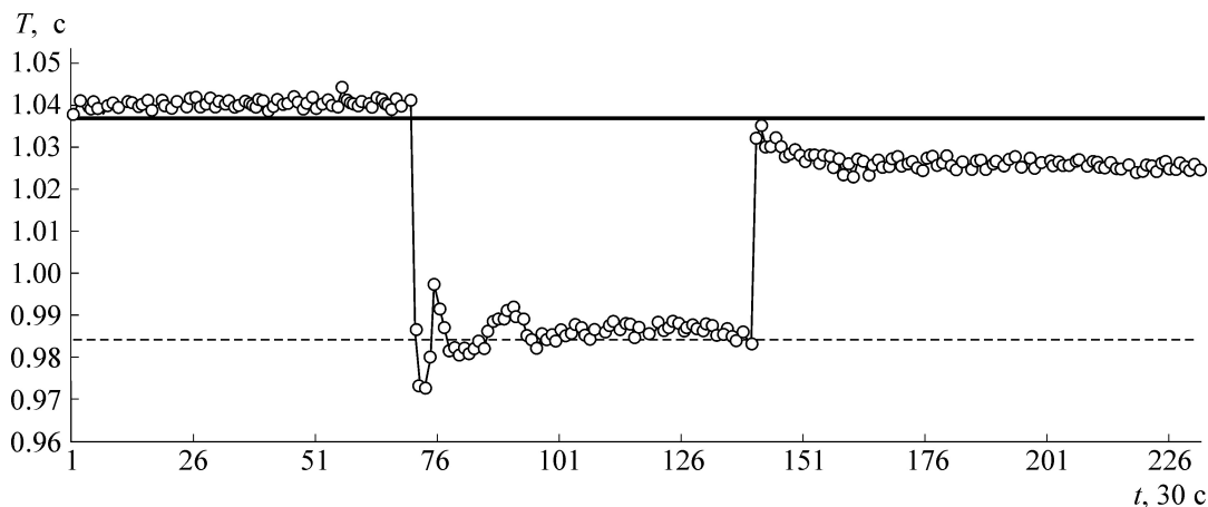
Рис. 11. Одиночный выброс – обратимый дискретный переход между соседними уровнями УСУП в дальнейшем ходе многосуточного мониторинга, представленного на рис. 10 (ср. с рис. 56).
