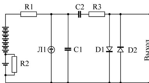
Рис. 2. Принципиальная схема релаксационного генератора на неоновой лампе Л1.
