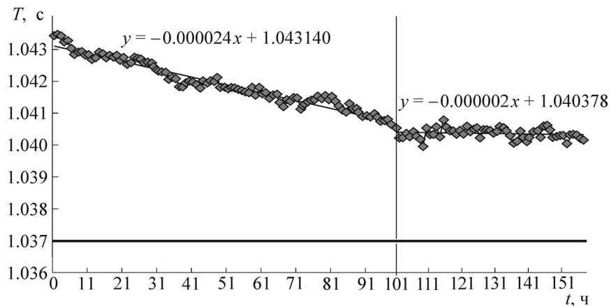
Рис. 10. Результат мониторинга периода RC-генератора в близкой окрестности T_{-20;0} = 1,037 с. Возможной причиной наблюдения универсальной системы утраивающихся периодов для дрейфующих значений периода может оказаться феномен их стабилизации в окрестностях уровней T_{k;m} .
