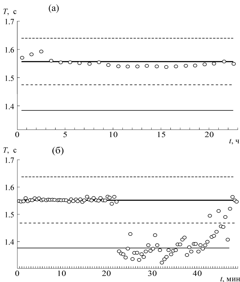
Рис. 5. (а) – Итог суточного мониторинга периода RC-генератора в окрестности периода T_{-19;1} = 1,555 с. Толщина горизонтальных линий, которые представляют уровни УСУП, качественно отвечает вероятности их наблюдения, которая, согласно накопленной эмпирике, быстро падает с ростом абсолютной величины параметра m периода T_{k;m} . На рисунке представлены четыре уровня – маловероятные, T_{-24;-7} = 1,639 с и T_{-14;9} = 1,476 с (штриховые линии), весьма вероятный, T_{-19;1} = 1,555 с (жирная линия) и несколько менее вероятный, T_{-21;-2} = 1,383 с (сплошная более тонкая линия). Общую картину уровней УСУП в окрестности этой зоны периодов см. ниже на рис. 14 и 15. (б) – Обратимый переход между уровнями УСУП T_{-19;1} = 1,555 с и T_{-21;-2} = 1,383 с на заключительном этапе суточного опыта, представленного на рис. 5а. Переход произошел в окрестности момента почти точного совпадения периода RC-генератора с периодом УСУП. RC-генератор находился в течение опыта в кожухе, несколько демпфирующем изменения температуры в лаборатории.
