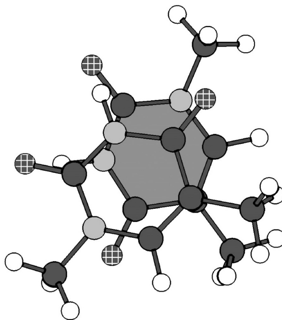
Рис. 4. Схема взаимного положения двух молекул 1-метилтимина для минимума «стекинг 2».
