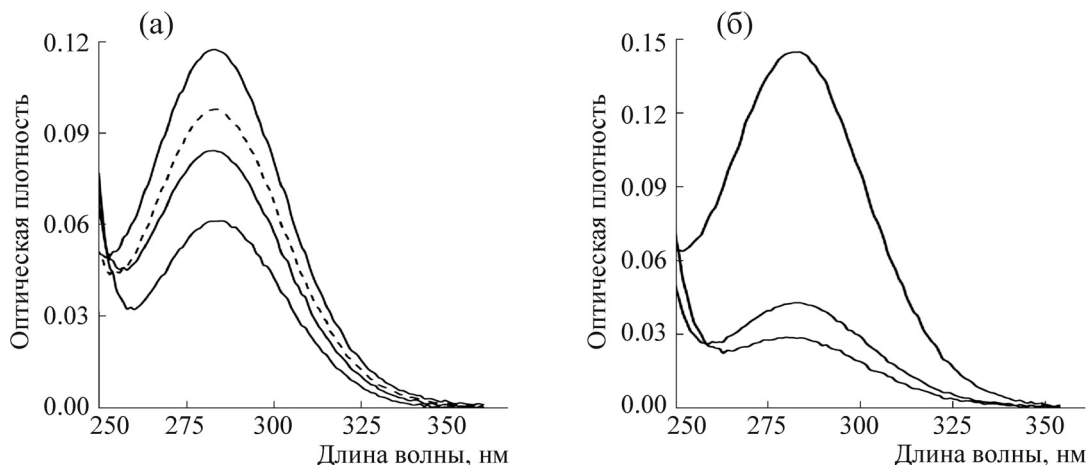
Рис. 10. Спектры поглощения дитиандра, образующегося из дитиотреитола (0,75 мМ) в присутствии метионина в реакции с N-ацетил-N-хлор-2,2-диметилтаурином (рН 5,6) или N,N-дихлор-2,2-диметилтаурином (рН 5,25). (а) – Исходная концентрация N-ацетил-N-хлор-2,2-диметилтаурина 0,424 мМ, а концентрации метионина 0, 5, 10 и 20 мМ (кривые по порядку сверху вниз). (б) – Исходная концентрация N,N-дихлор-2,2-диметилтаурина 0,255 мМ (концентрация активного хлора 0,51 мМ), а концентрации метионина – 0, 10 и 20 мМ (кривые по порядку сверху вниз).
