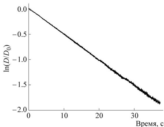
Рис. 9. Кинетика убыли N,N-дихлор-2,2-диметилтаурина (0,25 мМ) при взаимодействии с метионином (10 мМ) в режиме реакций первого порядка (рН 5,26). D_0 и D – оптическая плотность в начальный и текущий моменты.
