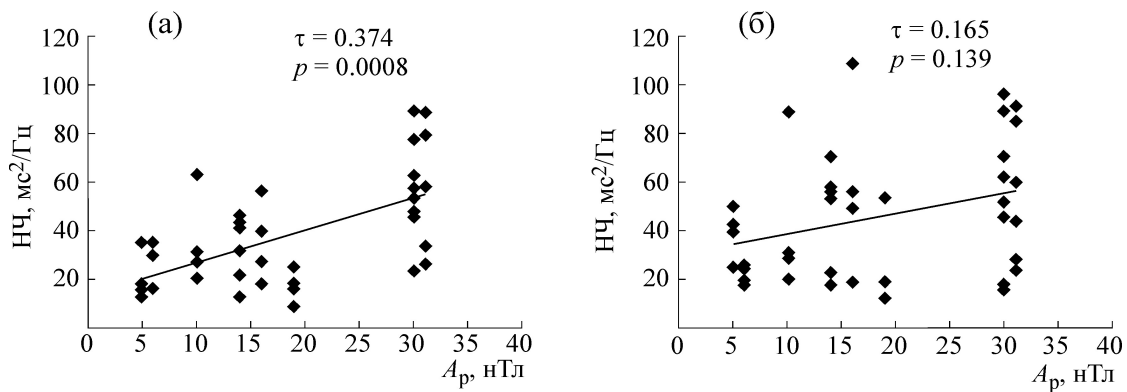
Рис. 3. Влияние геомагнитной активности на низкочастотный компонент variability сердечного ритма в условиях естественного (а) и экранированного (б) геомагнитного поля. \tau – Коэффициент корреляции Кендалла, p – значимость корреляции.
