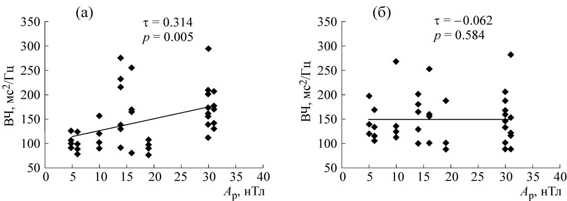
Рис. 4. Влияние геомагнитной активности на высокочастотный компонент variability сердечного ритма в условиях естественного (а) и экранированного (б) геомагнитного поля. \tau – Коэффициент корреляции Кендалла, p – значимость корреляции.
