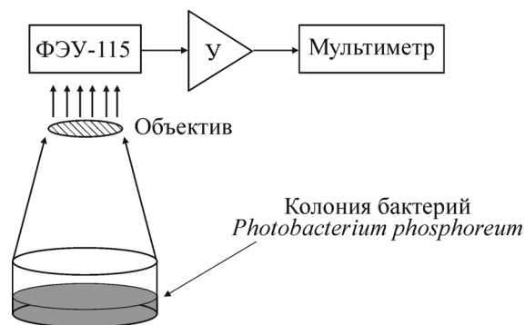
Рис. 1. Блок-схема экспериментальной установки. Пояснения в тексте.
